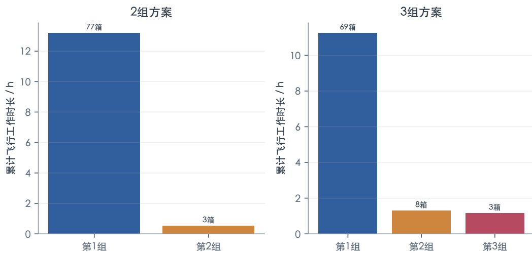
图 8-3 两组与三组方案的累计运输任务时长对比
