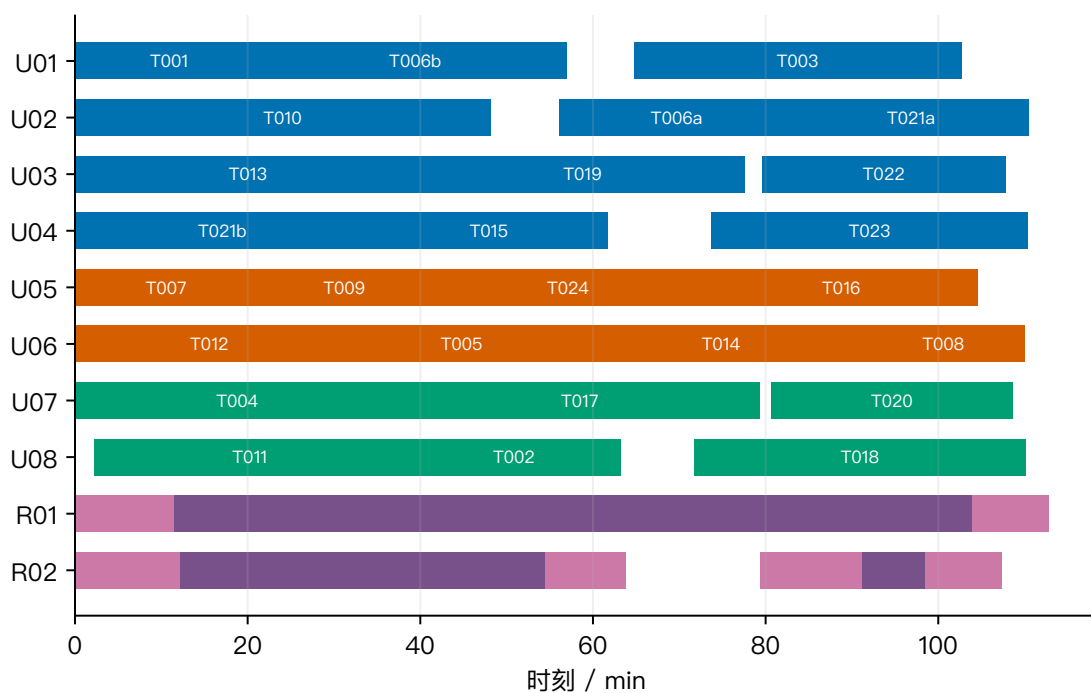
图 7: 主方案运输与中继架次时间表
