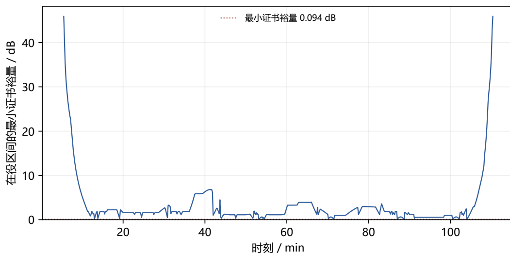
图 7-4 连续通信证书裕量的时间下包络
