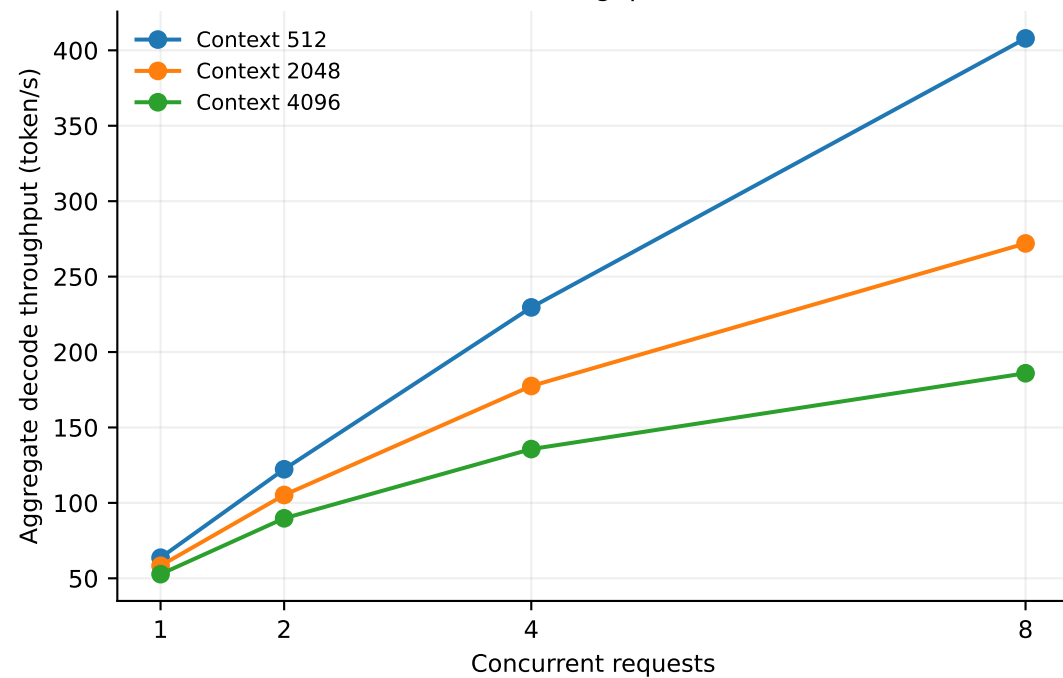
(d) Decode throughput saturation
