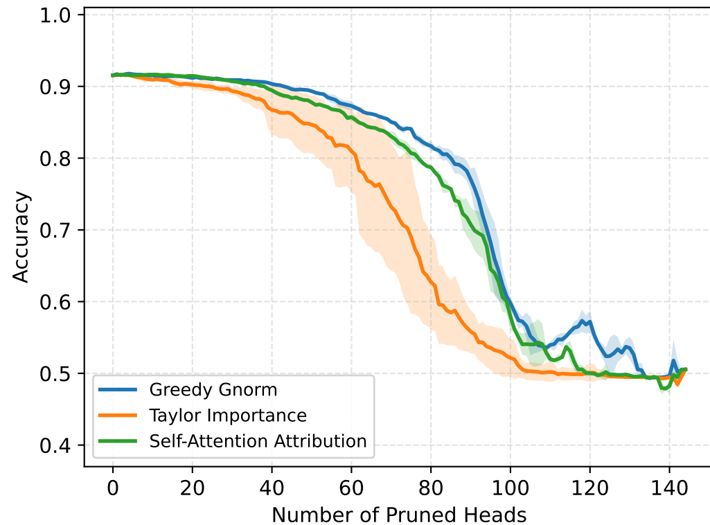
QNLI
