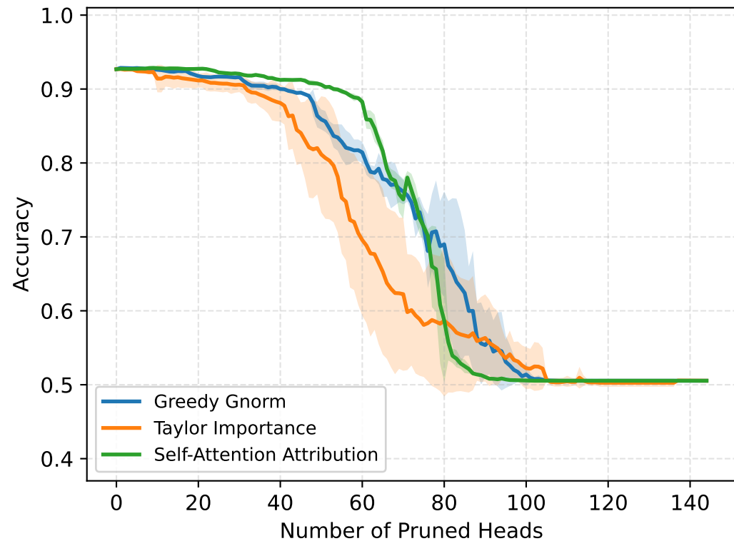
QNLI
