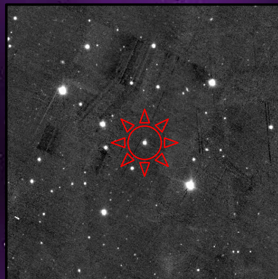
FOV of LAMOST J1327 ( PanSTARRS-1 )
