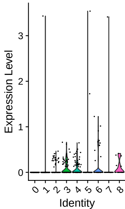
NRAS
