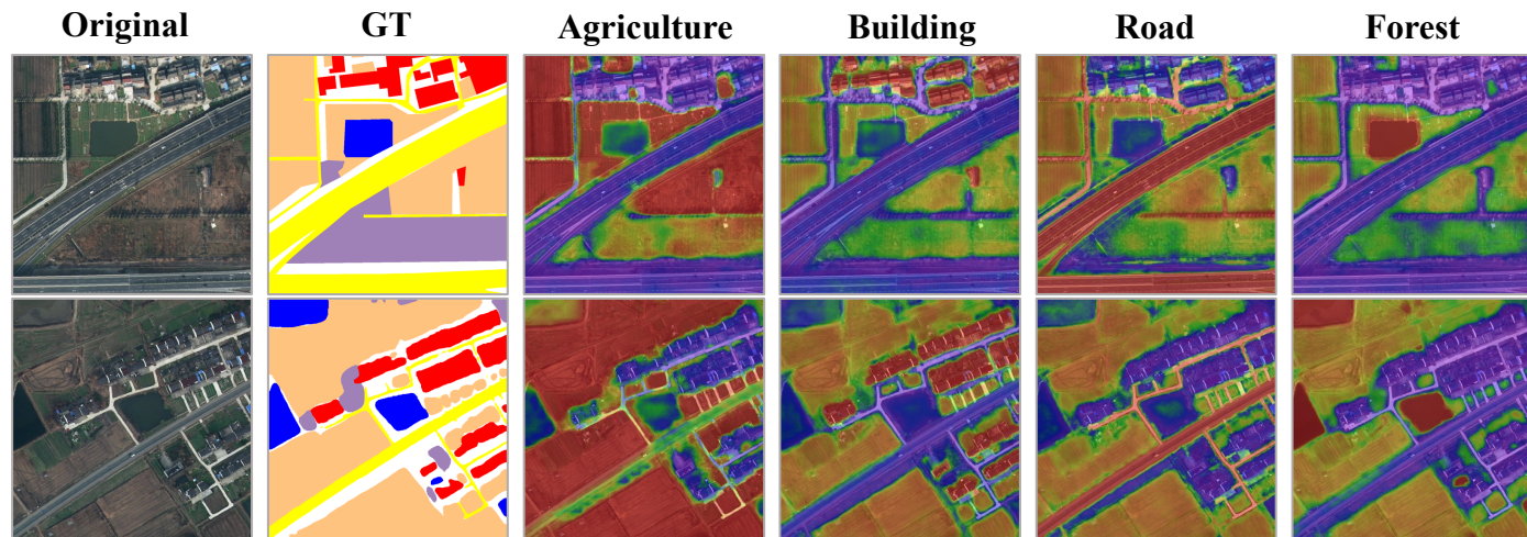
LoveDA
