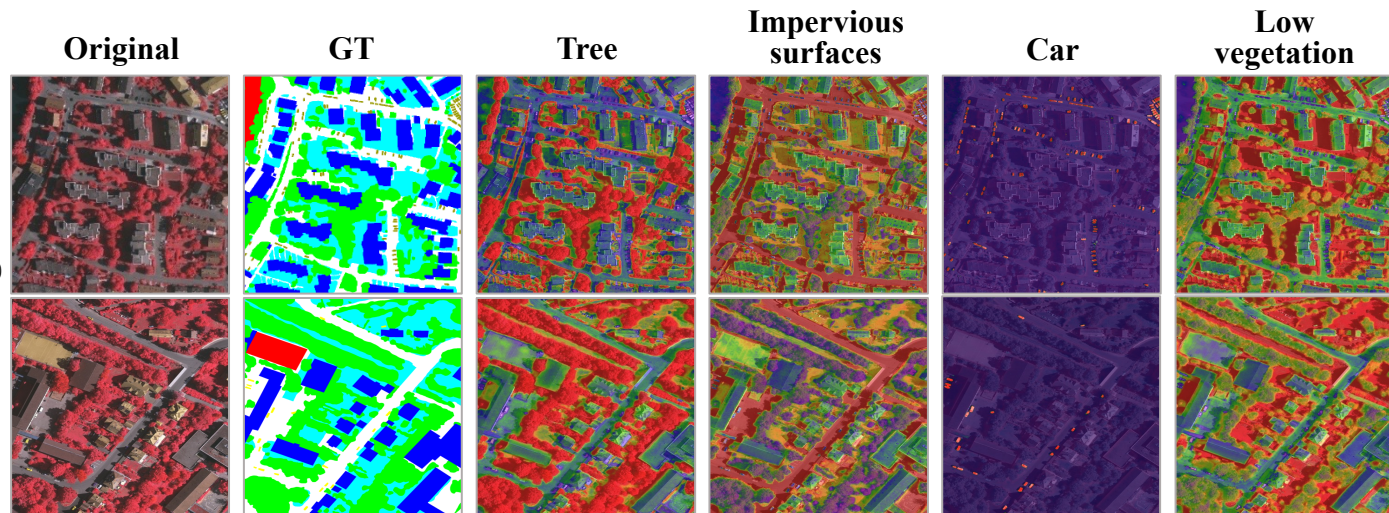
Vaihingen
