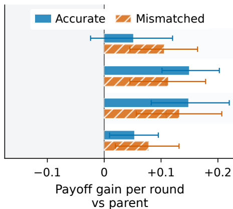
(d) S3: Thinking ON
