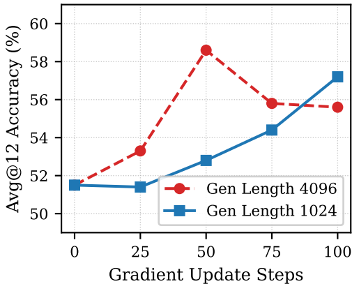
AIME24 (Qwen3-1.7B)
