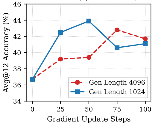
AIME25 (Qwen3-1.7B)
