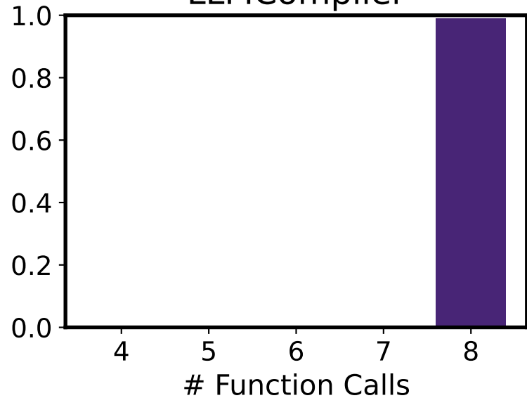
LLMCompiler
