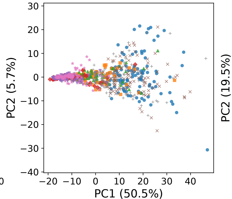
B t-STDP
