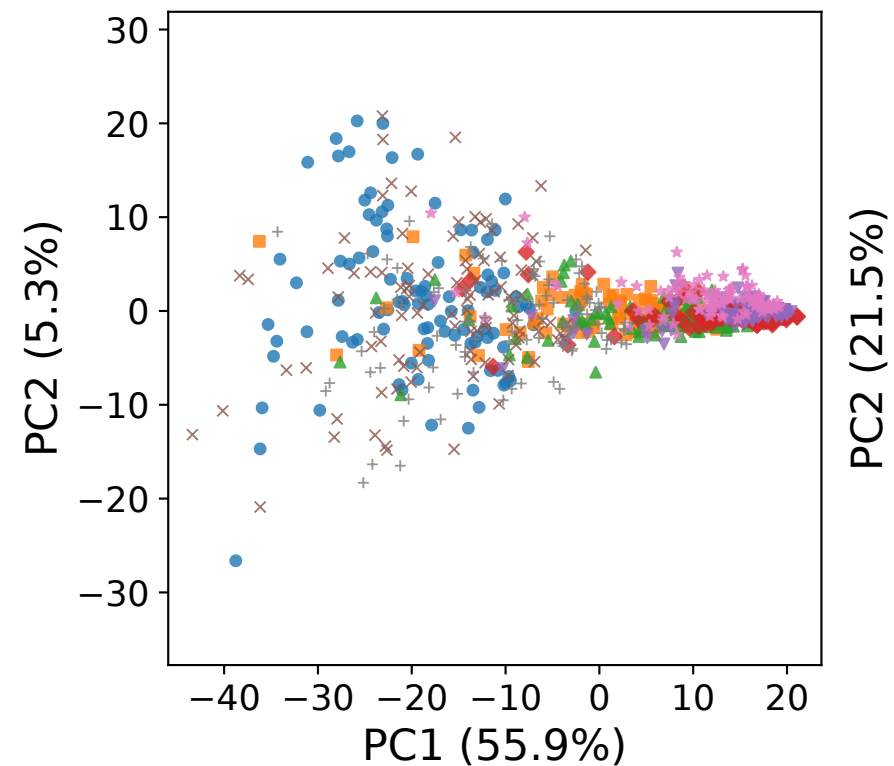
B t-STDP
