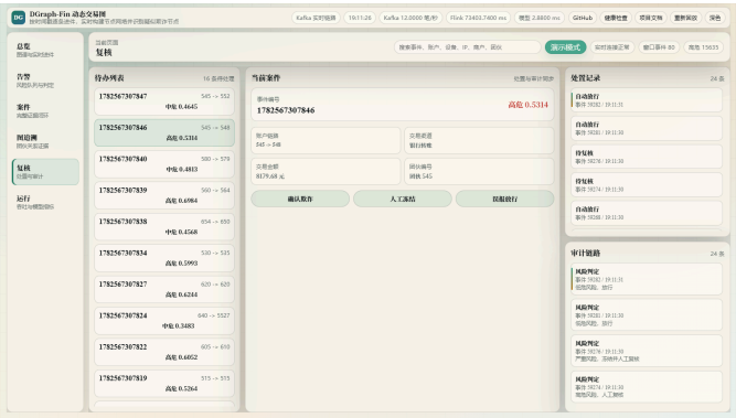
图 10 复核结果与审计留痕
