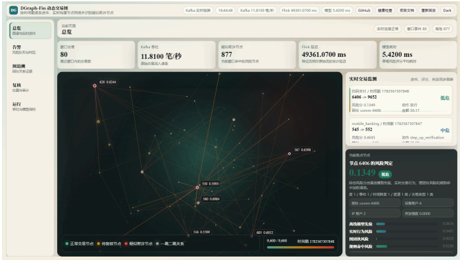
图 9-1 实时交易监测与运行指标
