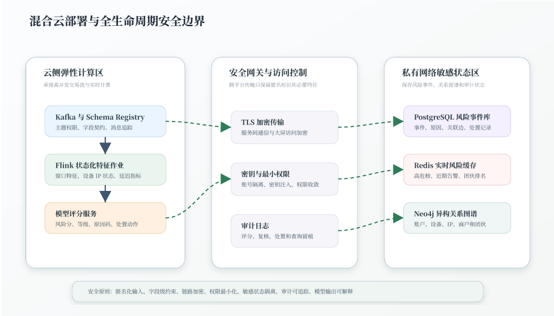
图 11 混合云部署与全生命周期安全边界：云侧承接弹性流处理，私有网络保存风险事件、图谱和审计状态。
