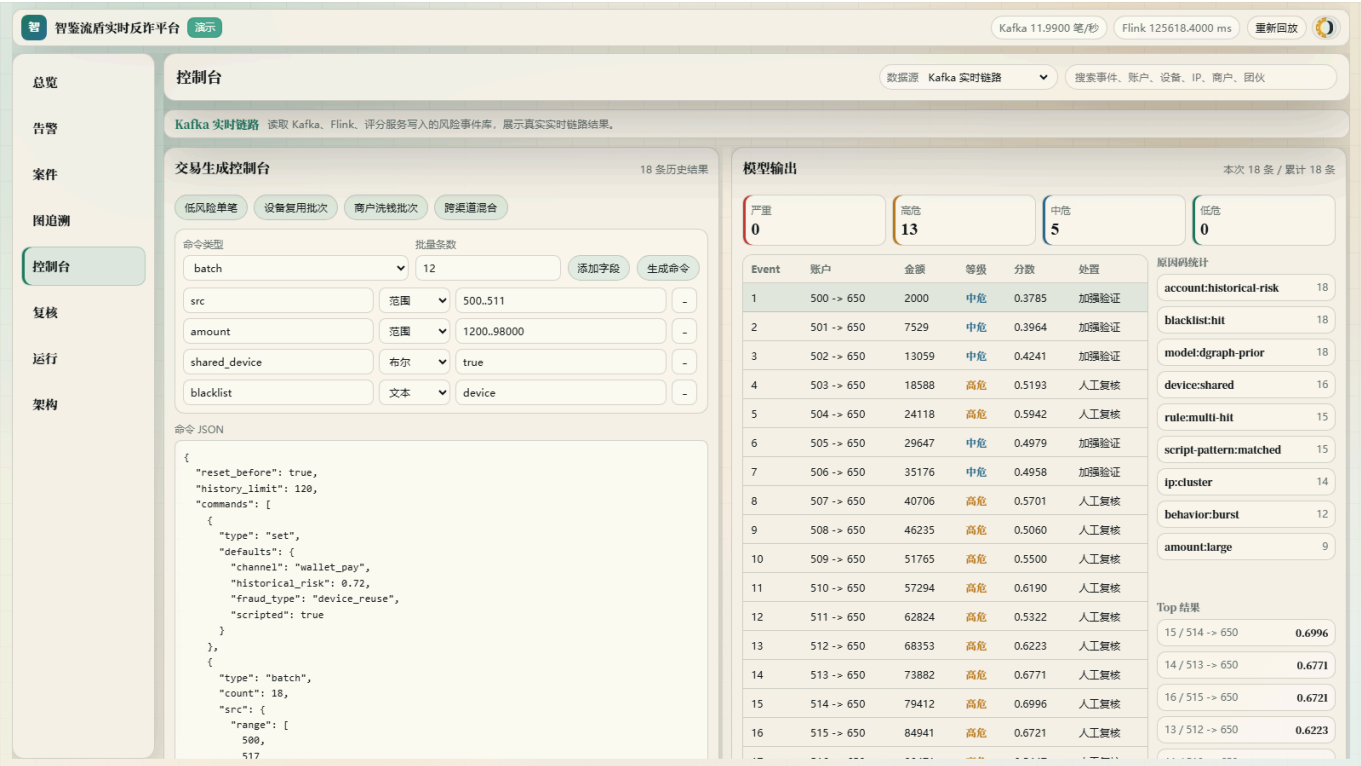
图 8 前端交易生成控制台：左侧构造仿真交易流，右侧同步展示模型输出、原因码统计、Top 风险结果和处置建议。
