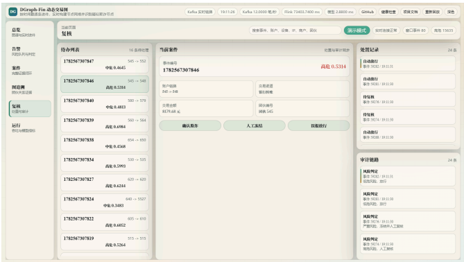
图 9-4 复核结果与审计留痕
