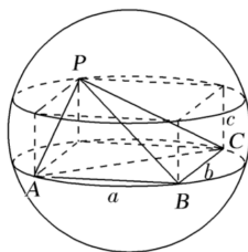
图 3.1: 三棱锥的外接球就是长方体的外接球
