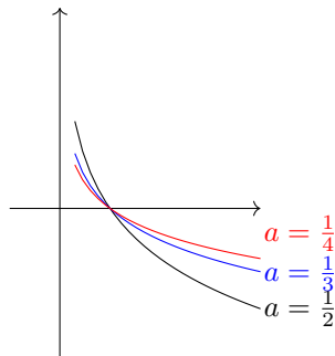
图 6.10: a < 1 ，函数单调减
