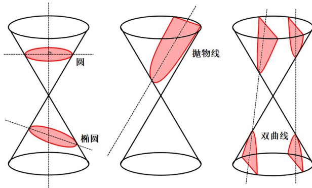
图 15.1: 被斜切得到的三种曲线
