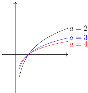
图 6.9: a > 1 ，函数单调增
