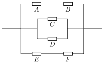
图 34.1: 题 34.1 的系统图
