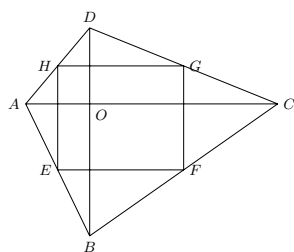
图 7.43: 对角线垂直的四边形
