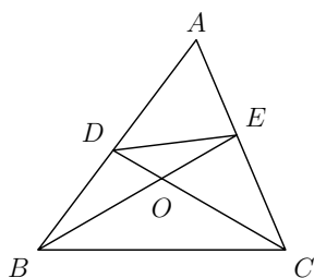
图 7.4: 三等角四边形
