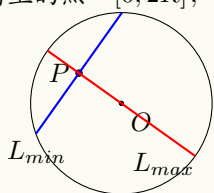
过圆内点的弦长范围
