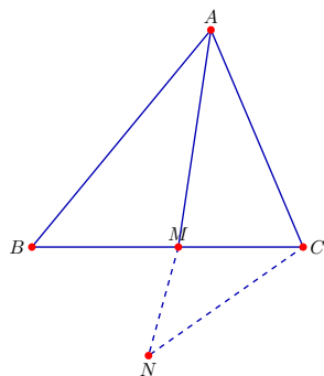
图 9.22: 角平分线定理
