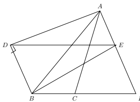
图 7.31: 练习图
