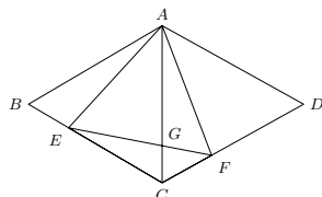
图 7.50: 含 60^\circ 度角的菱形
