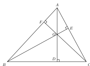
图 9.47: 三角形的垂心
