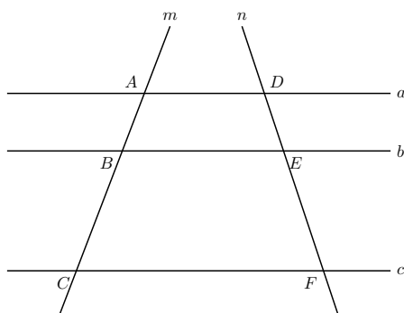
图 9.4: 平行线分线段成比例
