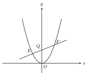
图 11.1: 二次函数与角平分线
