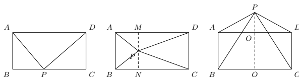
图 7.42: 矩形勾股定理
