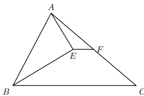
图 7.121: 练习图
