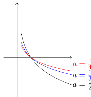
图 19.10: a < 1 ，函数单调减
