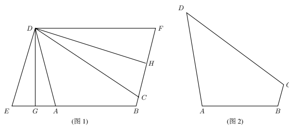
图 7.3: 三等角四边形
