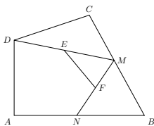
图 7.93: 练习图
