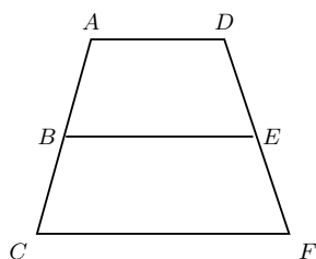
图 9.9: 梯形中的比例线段
