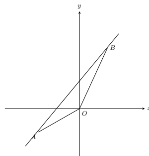
图 5.4: 有一个顶点在原点的三角形
