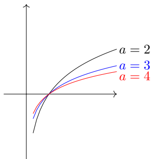
图 19.9: a > 1 ，函数单调增
