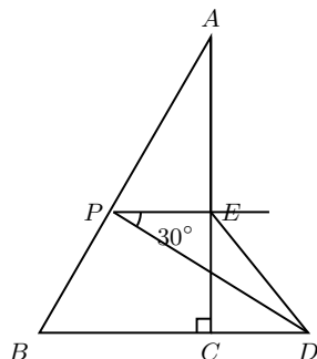
图 7.108: 练习图
