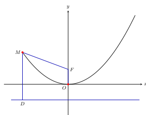
图 11.3: 抛物线的焦点与准线
