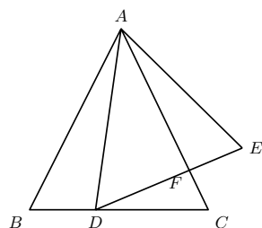
图 9.52: 练习图
