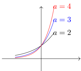
图 19.6: a > 1 ，函数单调增
