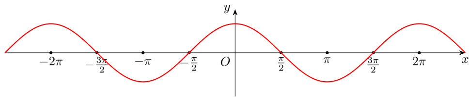
图 21.3: y = \cos x 的函数图像
