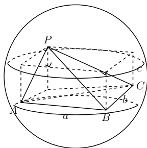
图 24.1: 三棱锥的外接球就是长方体的外接球
