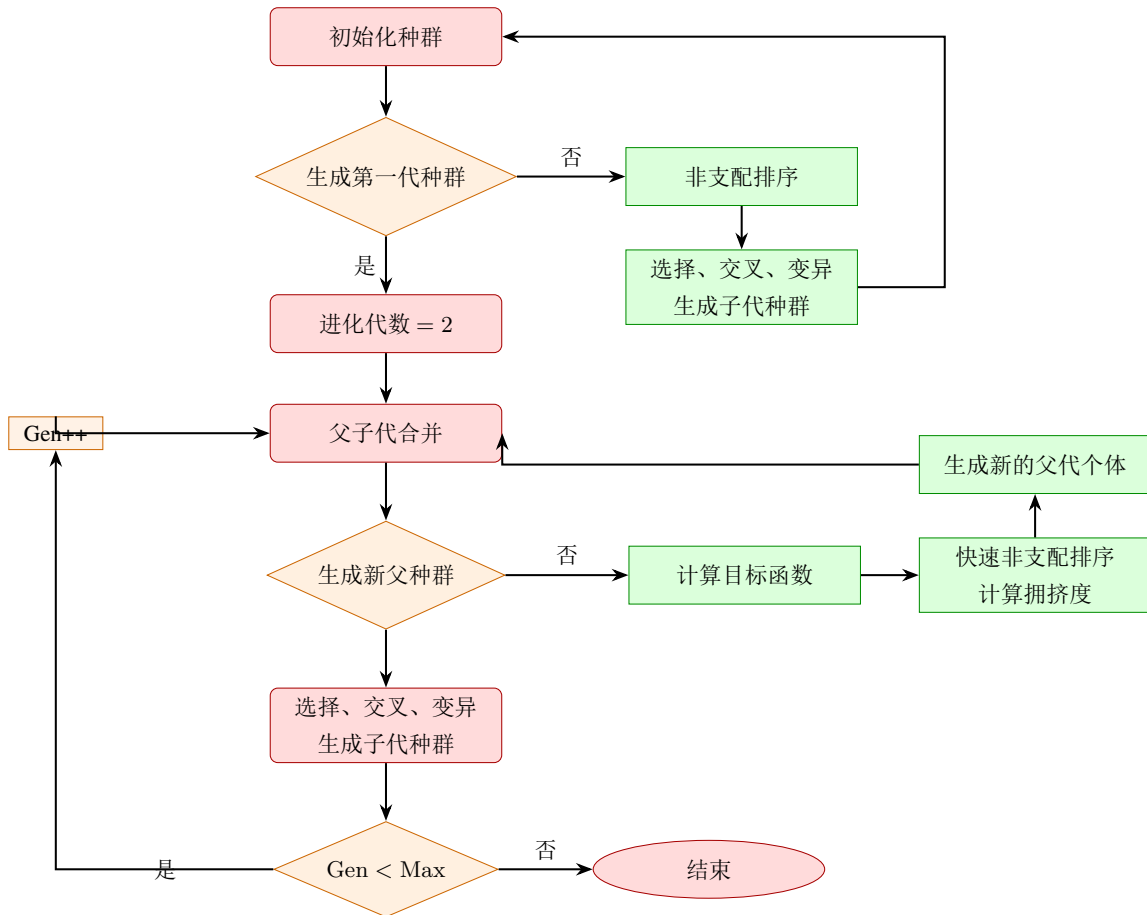
图 53.1: NSGA-II 算法流程图
