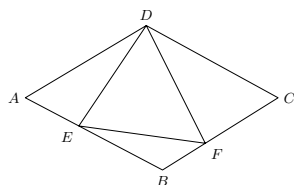
图 7.51: 练习图
