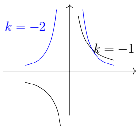
图 19.3: k 为负整数
