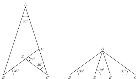
图 9.1: 黄金三角形
