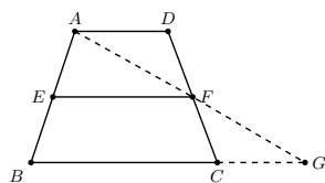
图 7.117: 梯形中位线
