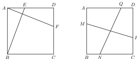
图 7.65: 十字架模型图
