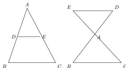
图 9.6: 三角形一边的平行线
