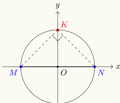
以 MN 为直径的圆中， K 处的圆周角为直角
