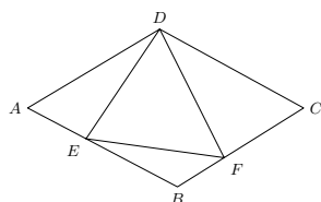
图 7.52: 练习图
