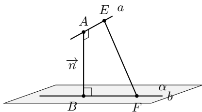
图 24.2: 异面直线公垂线段示意图
