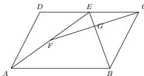
图 7.126: 练习图
