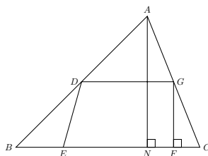
图 9.15: 三角形内接矩形
