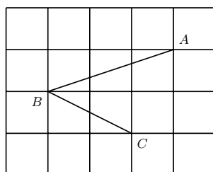
图 10.7: 45 度角模型
