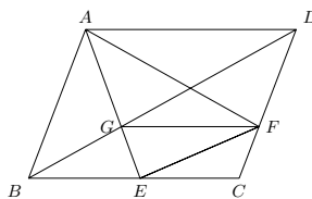
图 7.9: 练习图
