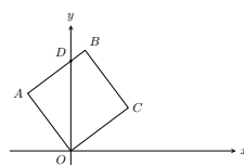
图 7.88: 练习图
