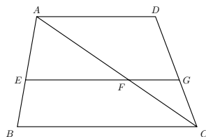
图 9.10: 练习图
