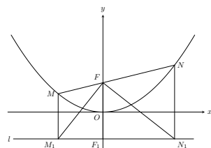
图 11.4: 抛物线与直角梯形
