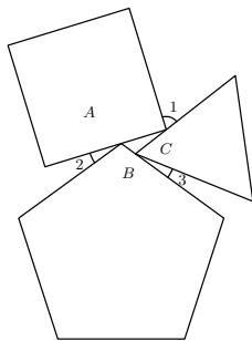
图 7.1: 正三角形、正方形与正五边形
