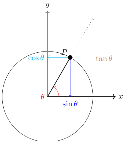
图 21.1: 三角函数线
