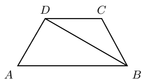
图 7.107: 有 60 度角的等腰梯形
