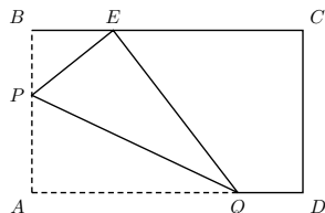
图 7.40: 练习图
