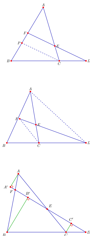
图 9.24: 梅涅劳斯定理
