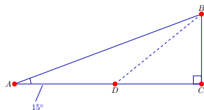
图 10.2: 15^\circ 度角的三角比计算
