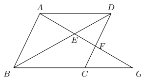
图 9.26: 练习图
