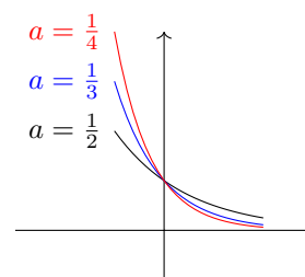
图 19.7: a < 1 ，函数单调减
