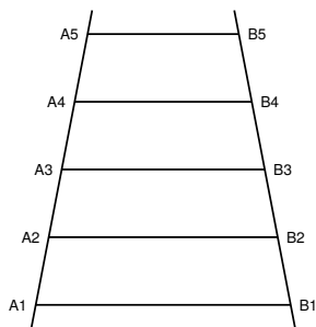
图 7.118: 等间距平行线
