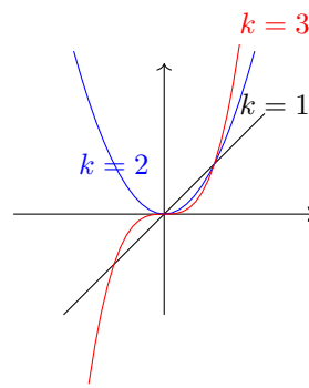
图 19.2: k 为正整数
