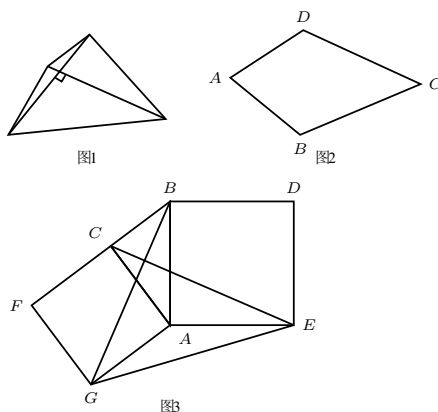
图 7.45: 练习图
