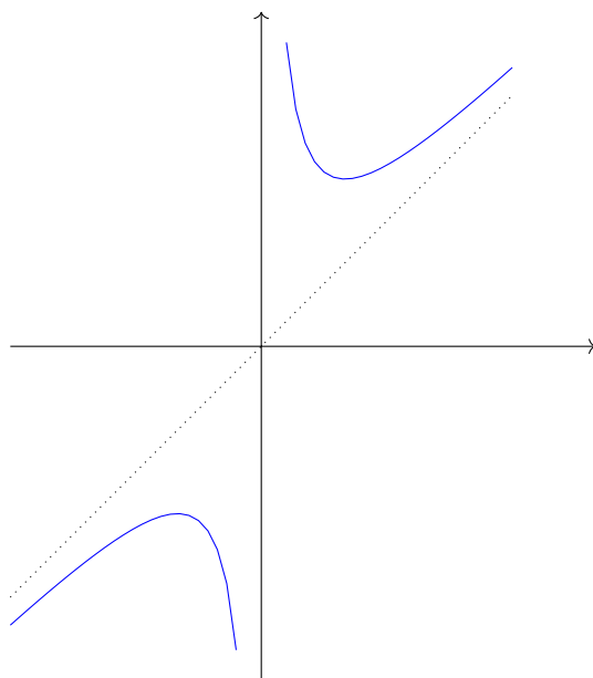
图 16.1: y = x + 1/x
