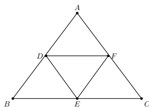
图 7.116: 三角形中位线
