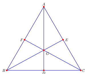
图 9.18: 三角形的重心
