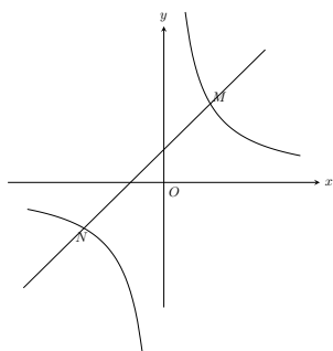
图 5.1: 一次函数与反比例函数
