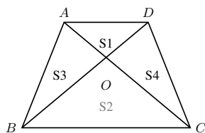
图 7.113: 蝴蝶定理模型图
