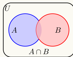
图 15.1: 定理韦恩图可视化
