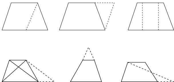
图 7.96: 梯形常见辅助线
