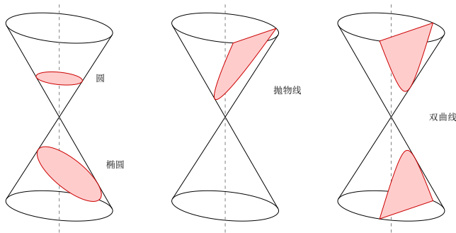
图 28.1: 被斜切得到的三种曲线
