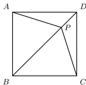
图 7.76: 对称模型
