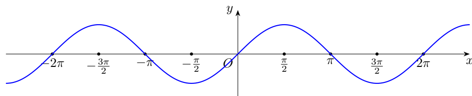
图 21.2: y = \sin x 的函数图像
