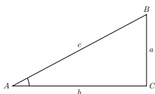
图 10.3: 解直角三角形
