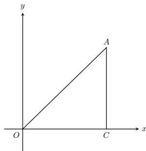
图 7.103: 练习图
