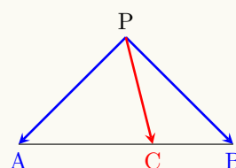
图 23.1: 定比分点示意图
