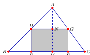
图 9.14: 三角形内接矩形
