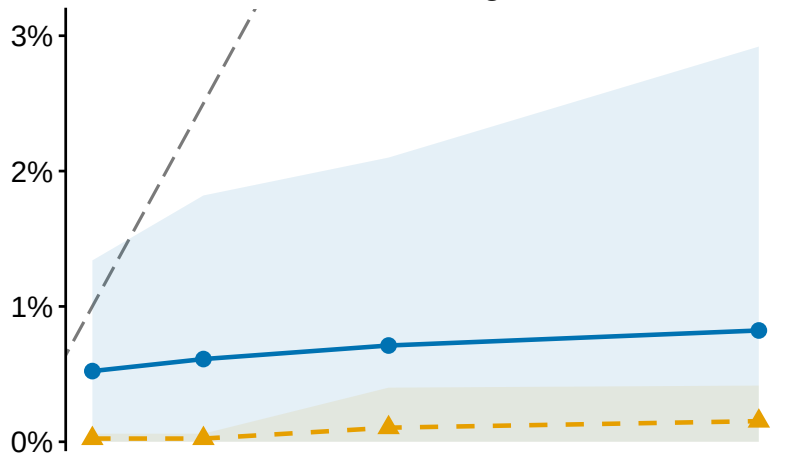
Linear designs
