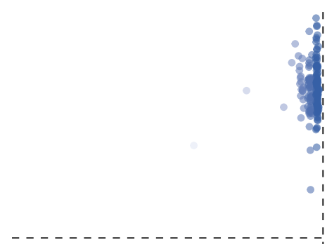
GPD
