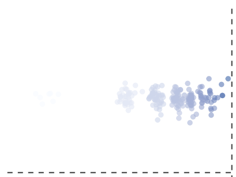
Pareto
