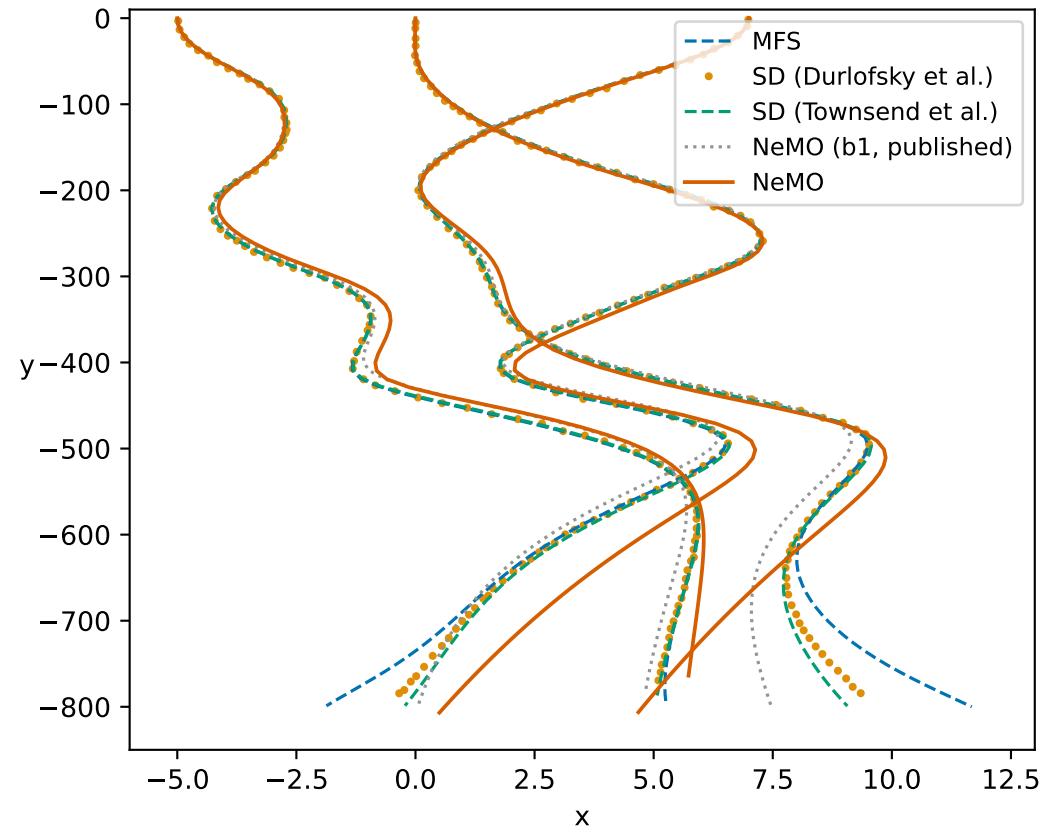
NeMO (moments pc8c + diag)
