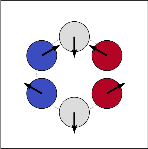
NeMO: M_{\circ} err 53 %, \Omega_z err 19 %, M_{\parallel} err 0.3 %
