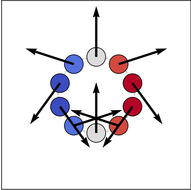
RPY: M_{\circ} err 143 %, \Omega_z err 35 %, M_{\parallel} err 2.9 %
