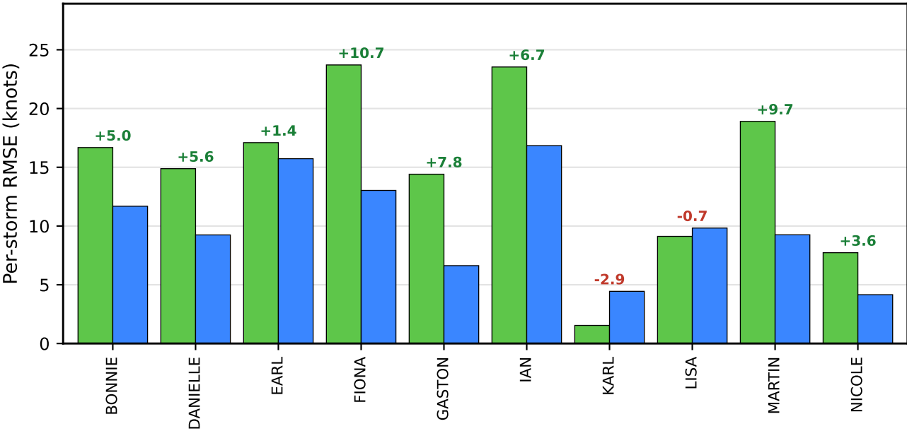
2022 (Validation)
