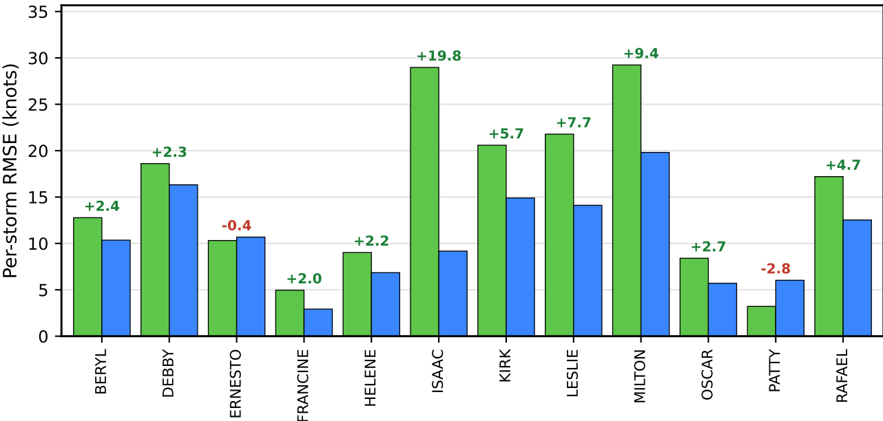
2024 (Test)
