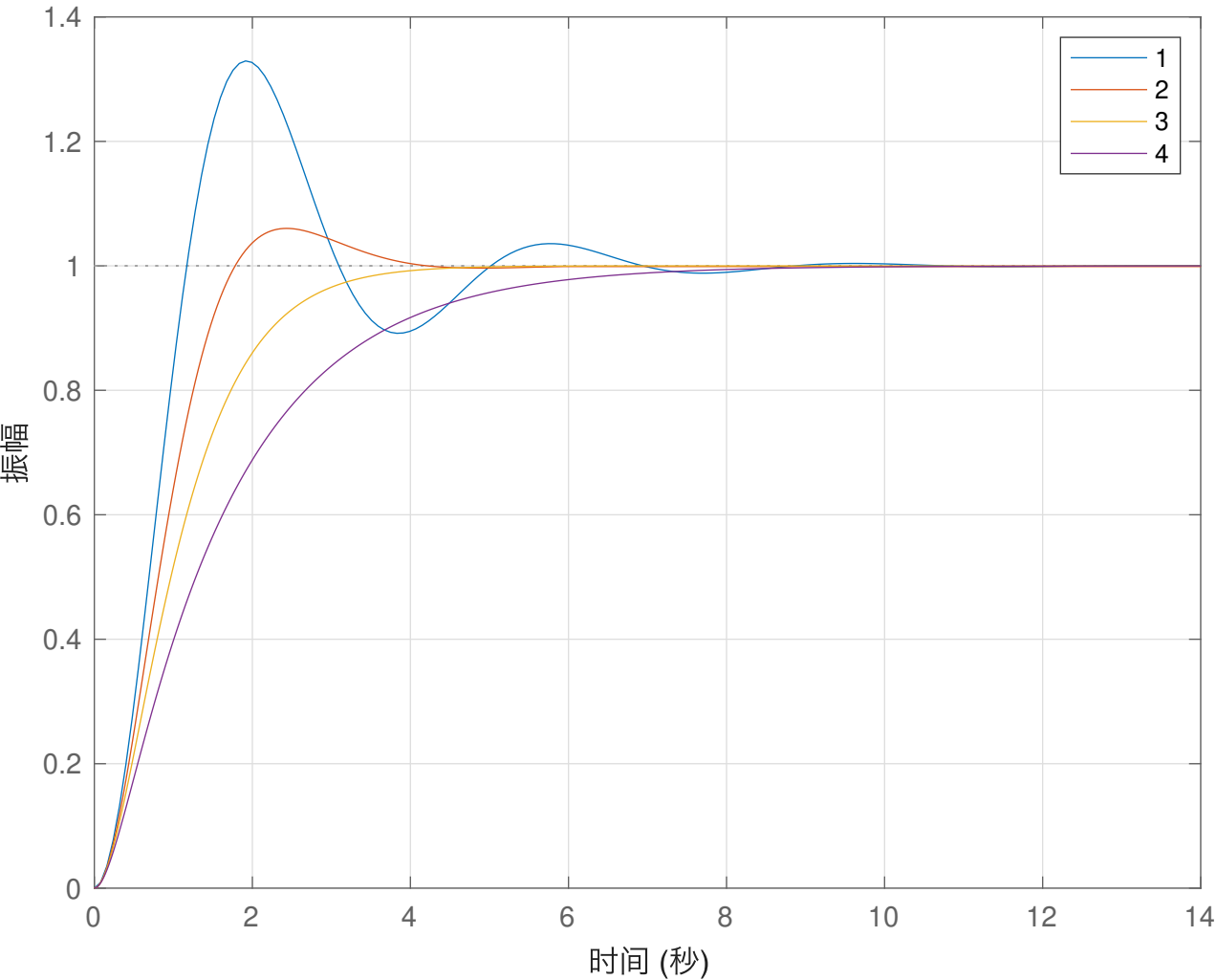
阶跃响应
