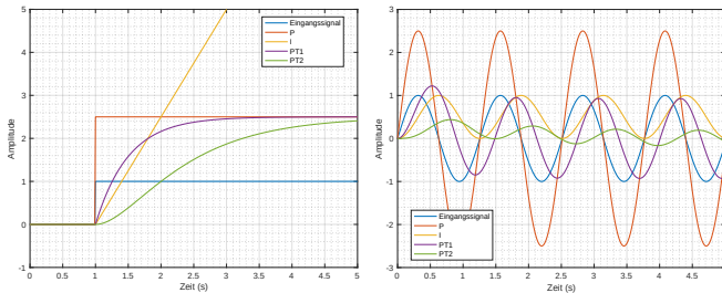
(a) 阶跃输入下的响应
