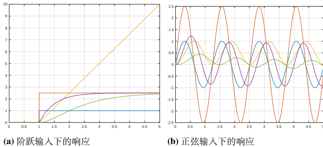
Abbildung 2: P、I、PT1 和 PT2 环节在不同输入信号下的输出比较
