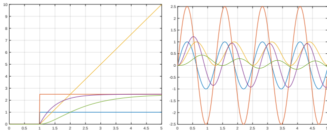
(a) 阶跃输入下的响应
