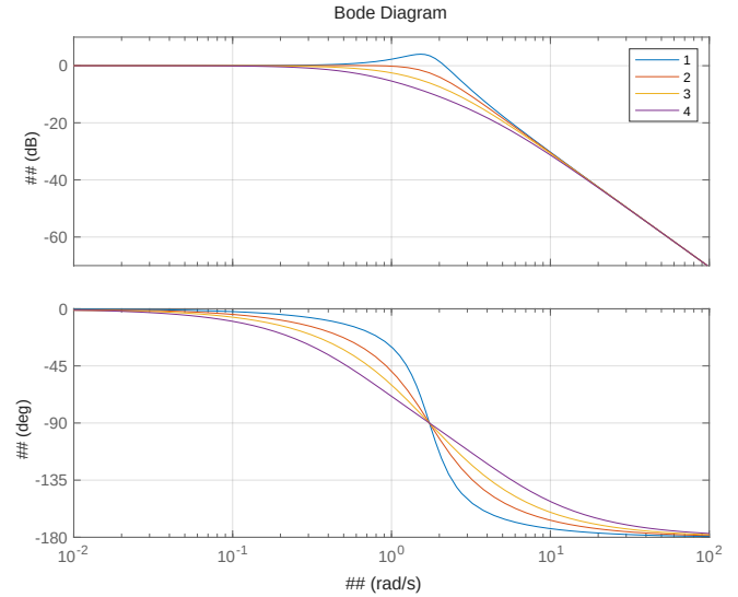
Abbildung 4: 固定固有频率、改变阻尼系数时 PT2 环节的 Bode 图
