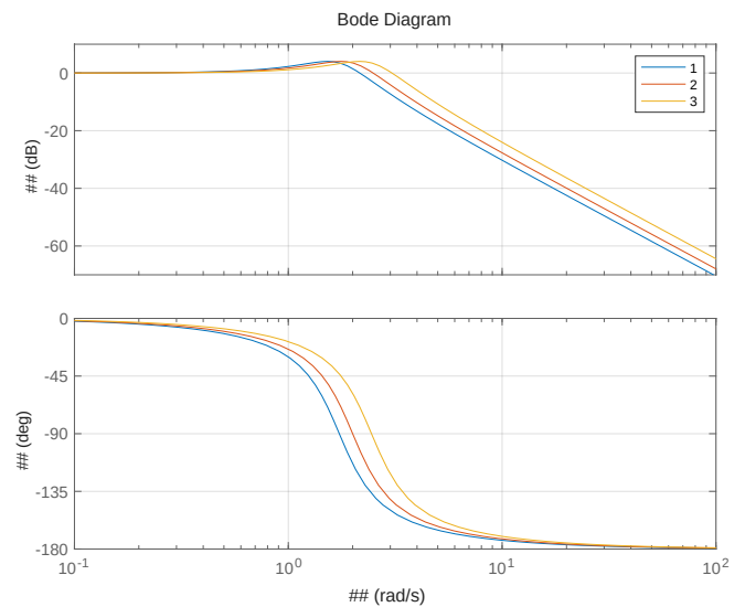
Abbildung 5: 固定阻尼系数、改变固有频率时 PT2 环节的 Bode 图
