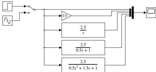
Abbildung 1: 用于比较 P、I、PT1 和 PT2 环节阶跃响应的 Simulink 模型
