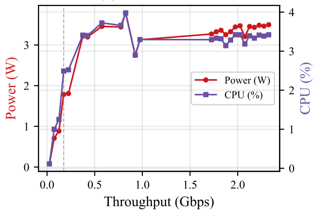
(d) Power and CPU
