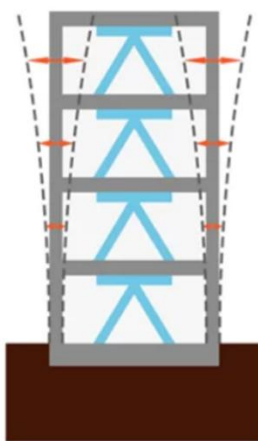
制震構造
