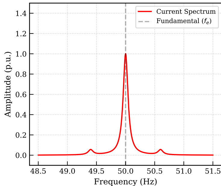
(d) Current Spectrum: 3P Sidebands
