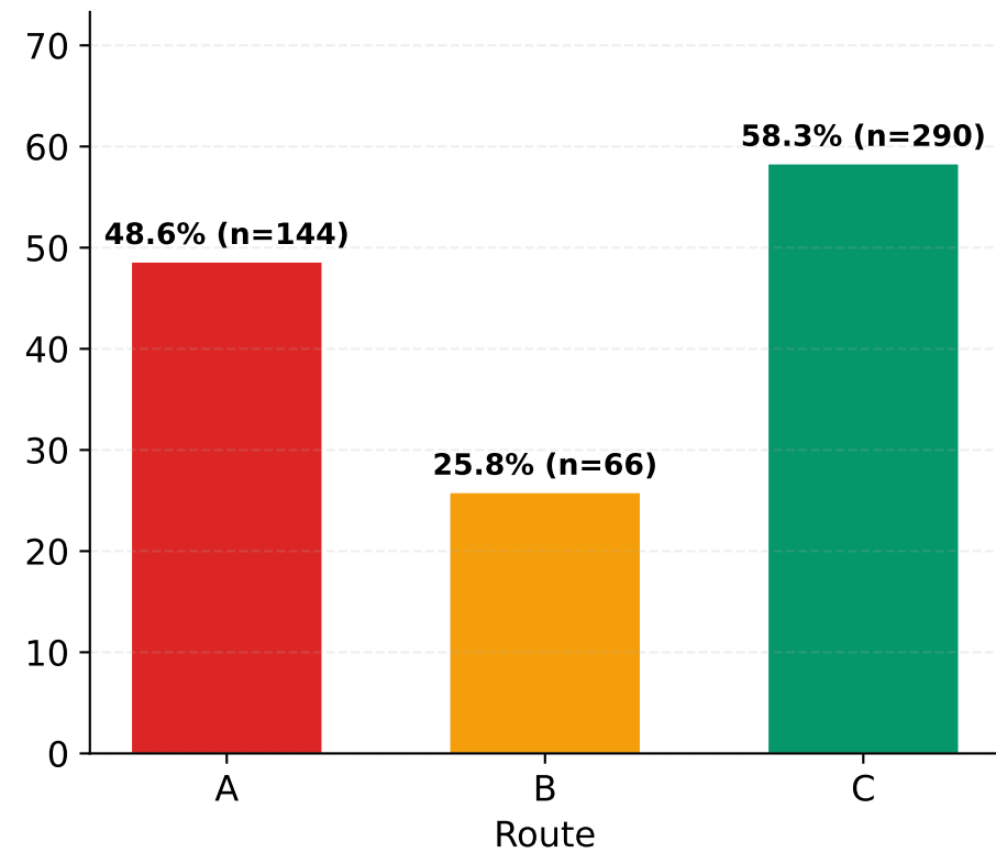
2WikiMHop
