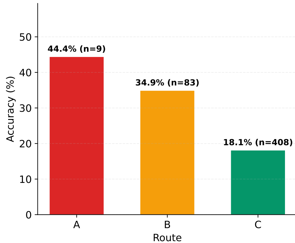
MuSiQue
