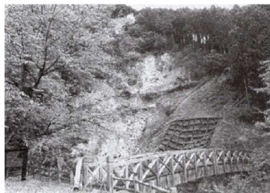
中央構造線露頭（飯高町月出）
