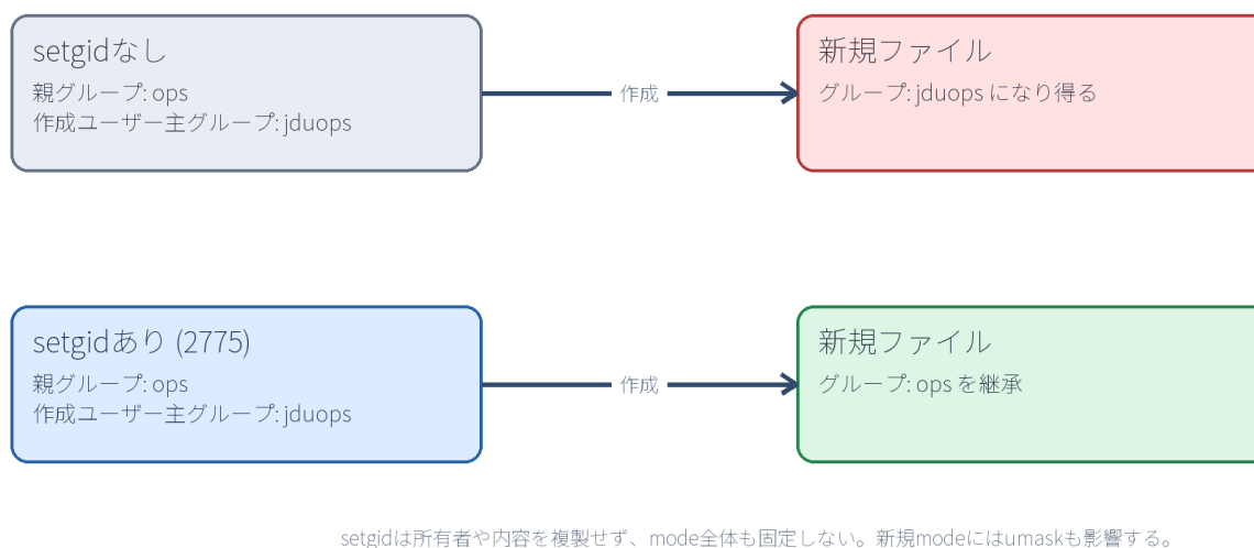
図7-2 setgid は新規項目の所有グループを親ディレクトリとそろえる。所有者、ファイル内容、アクセス権モード全体をコピーする機能ではない。
