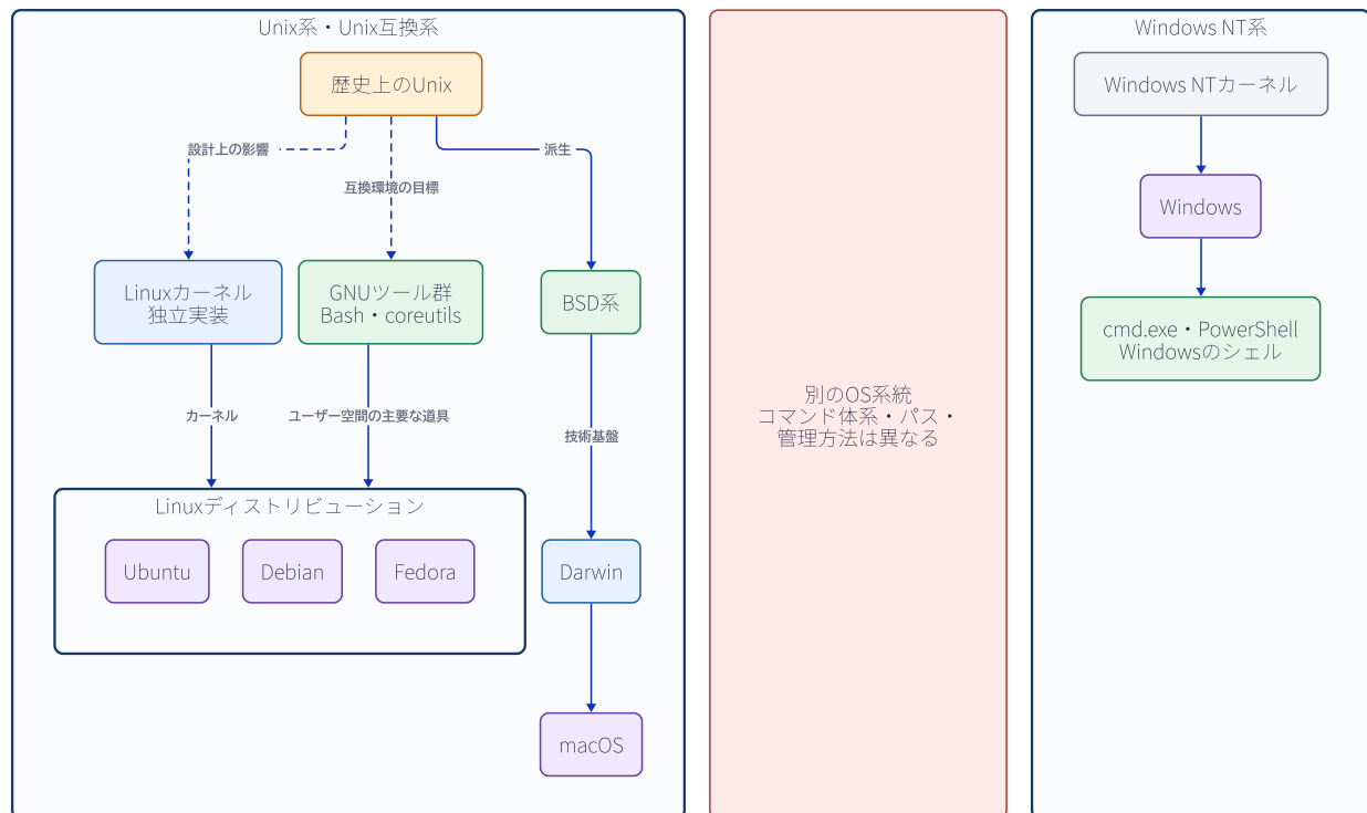
図2-1 Unix系・Unix互換系とWindows NT系は別の系統であり、コマンド体系の互換性を前提にできない。LinuxはUnixに似たインターフェースを持つ独立実装であり、macOSはLinuxの派生ではない。
