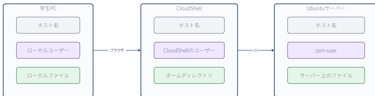
図1-4 各ホストは独立したOS環境を持ち、その中でユーザー、プロセス、ファイルが個別に管理される。
