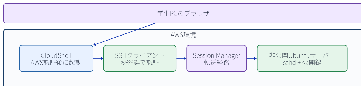
図12-1 AWS認証によってセッショントンネルを確立する層と、SSHがUbuntuユーザーを公開鍵認証する層は独立している。
