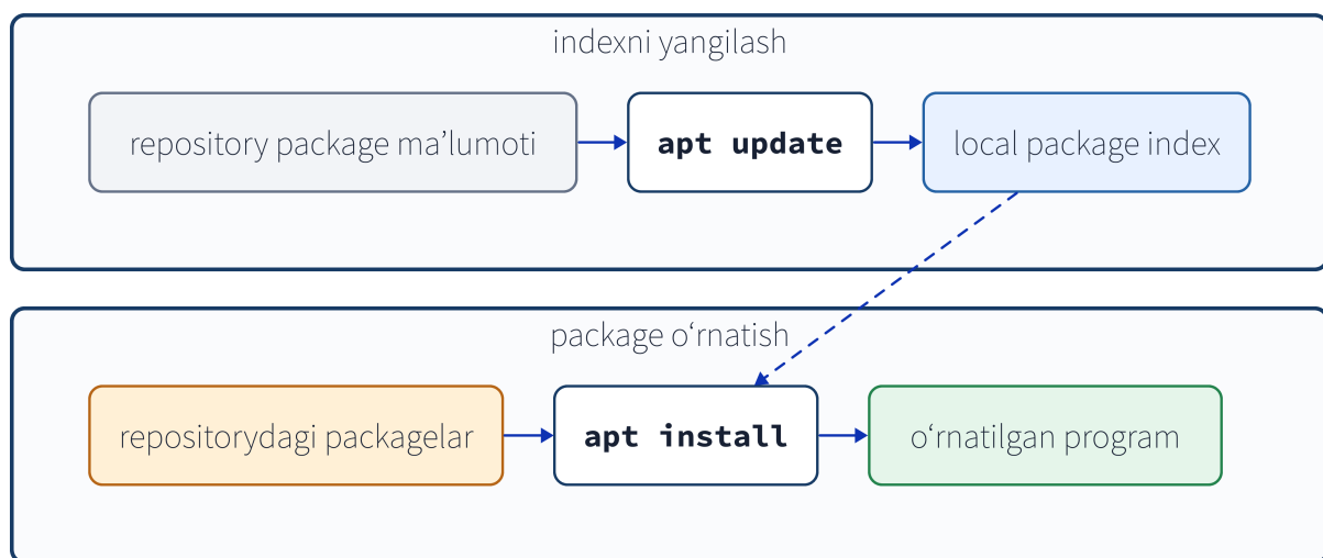
9-1-rasm. apt update mavjud pakagelar ro'yxatini yangilaydi; apt install esa package mazmunini olib o'rnatadi.
