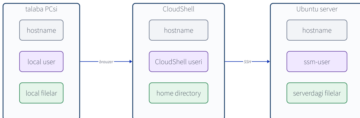
1-4-rasm. Har bir host alohida OS muhitiga ega; unda userlar , processlar va filelar mustaqil boshqariladi.
