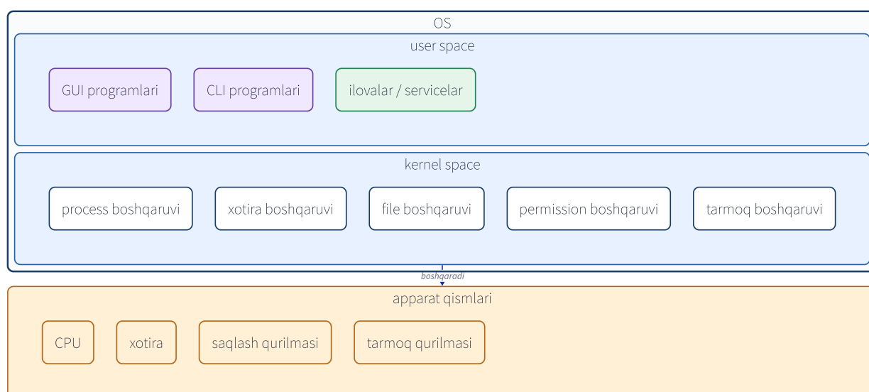
1-2-rasm. Keng ma'nodagi OS muhiti user space da ishlaydigan programlar va apparat qismlarini boshqaradigan kernel space dan iborat.
