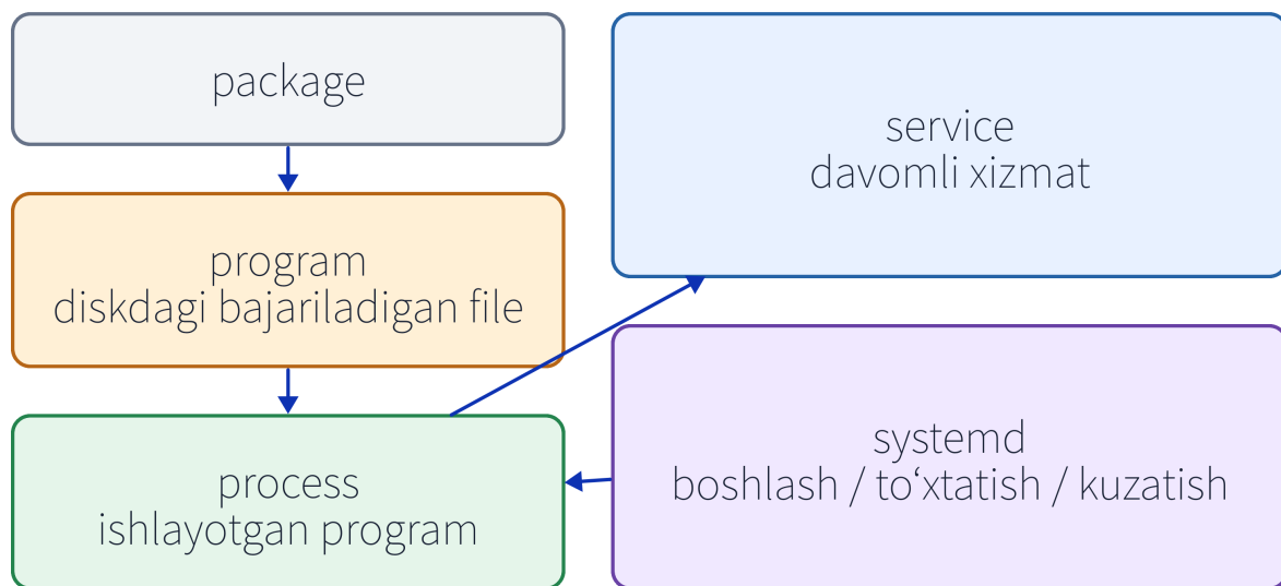
8-1-rasm. Saqlangan program, ishlayotgan process, boshqaruv birligi service va tarqatish birligi package alohida tushunchalardir.
