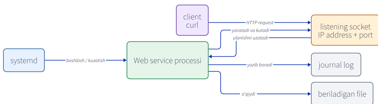
11-1-rasm. Boshqaruv (systemd), bajarish (process), aloqa (kernel va socket) hamda client requesti alohida vazifalardir. Bir service bir nechta socketga ega bo'lishi yoki umuman tarmoqdan foydalanmasligi mumkin.
