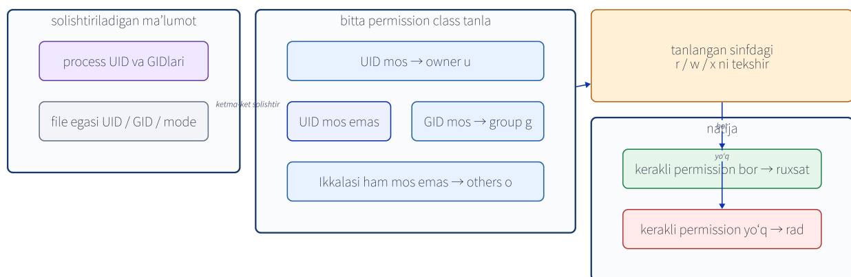
7-1-rasm. Process huquqlariga ko'ra u/g/o sinfi tanlanadi, keyin shu sinfdagi rwx belgilari amal mumkinligini aniqlaydi.
