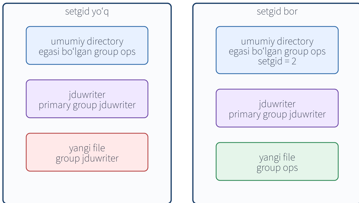
7-2-rasm. Setgid yangi obyektning groupini yuqori directory groupi bilan bir xil qiladi. U file egasi, mazmuni yoki butun permission modeni nusxalamaydi.
