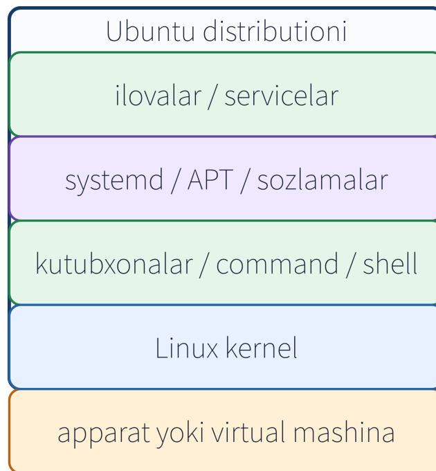
2-2-rasm. Distribution Linux kernel, kutubxonalar, asosiy commandlar, tizim boshqaruvi, packagelar va ilovalarni birlashtiradi. Bu tuzilma Ubuntu va Linuxni to'liq sinonim deb hisoblamaslikka yordam beradi.
