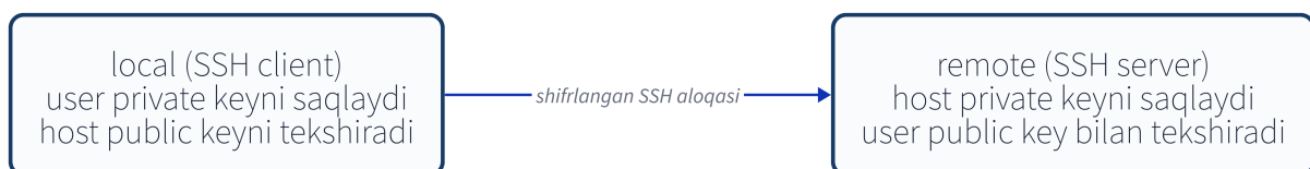
12-1-rasm. SSHda serverni aniqlaydigan host key va userni tasdiqlaydigan user key turli vazifani bajaradi.
