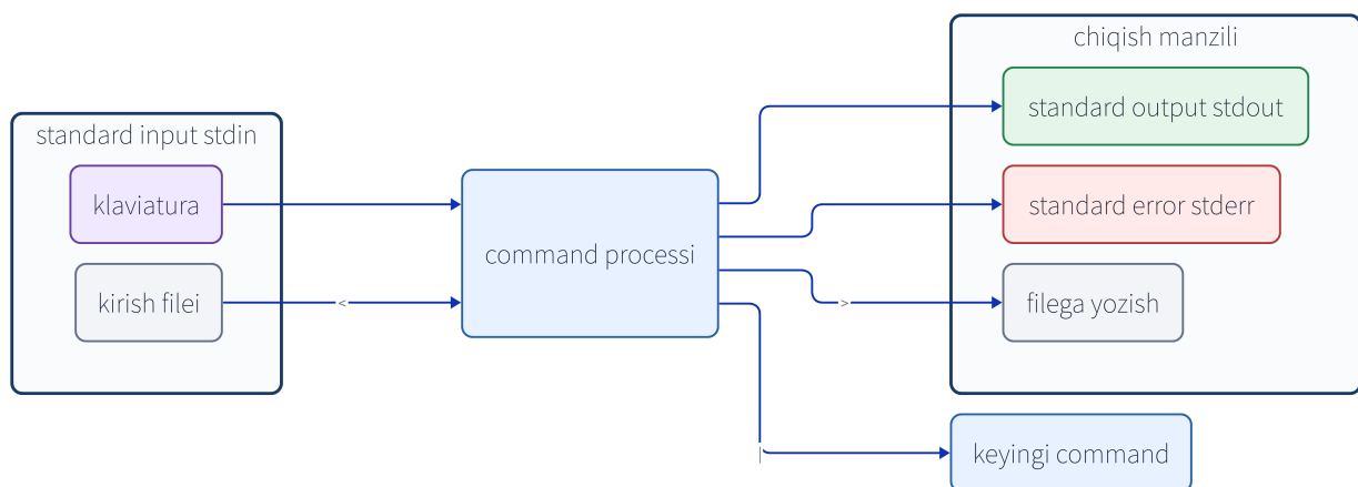
5-1-rasm. Programning uchta standart oqimi. > odatda stdout ni filega, | esa chapdagi commandning stdout ini o'ngdagi commandning stdin iga ulaydi.
