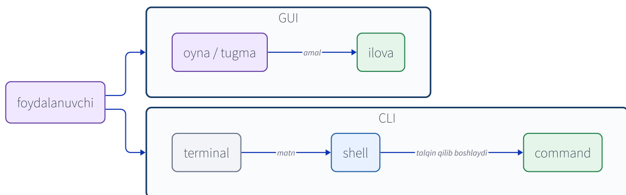
3-1-rasm. GUI va CLI parallel kirish usullaridir. CLI ishlatilganda terminal va shell vazifalarini farqlash kerak.
