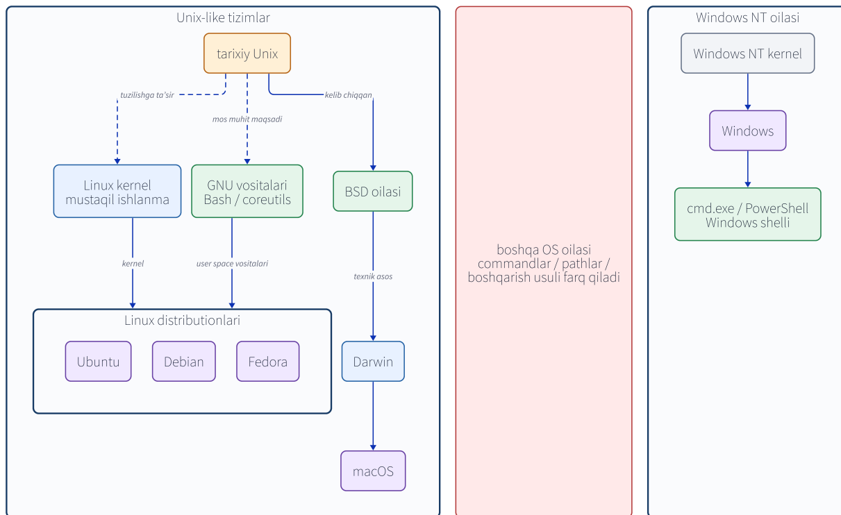
2-1-rasm. Unix-like va Unixga mos tizimlar Windows NT oilasidan alohida yo'nalishdir; ularning commandlari bir-biriga to'liq mos deb bo'lmaydi. Linux Unixga o'xshash interfacelarga ega mustaqil ishlanma, macOS esa Linuxdan kelib chiqmagan.
