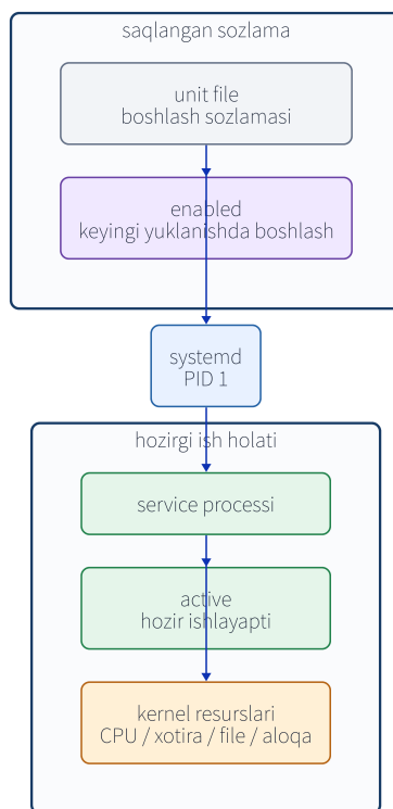
10-1-rasm. Unit — sozlama, systemd — boshqaruvchi, service processi esa haqiqiy ishni bajaruvchi.
