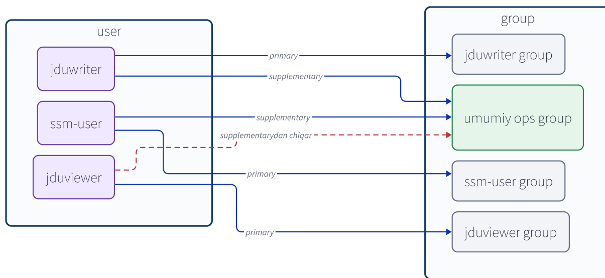
6-1-rasm. Har bir userning primary groupi va umumiy ishlash uchun qo'llanadigan supplementary grouplari o'rtasidagi munosabat.
