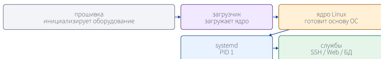
Рисунок 1-3. Ядро запускает первый процесс пространства пользователя; затем systemd запускает процессы служб в нужном порядке.
