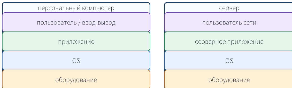
Рисунок 1-1. Несмотря на разное назначение и способы управления, ПК и сервер имеют общую основу: приложения, ОС и оборудование.
