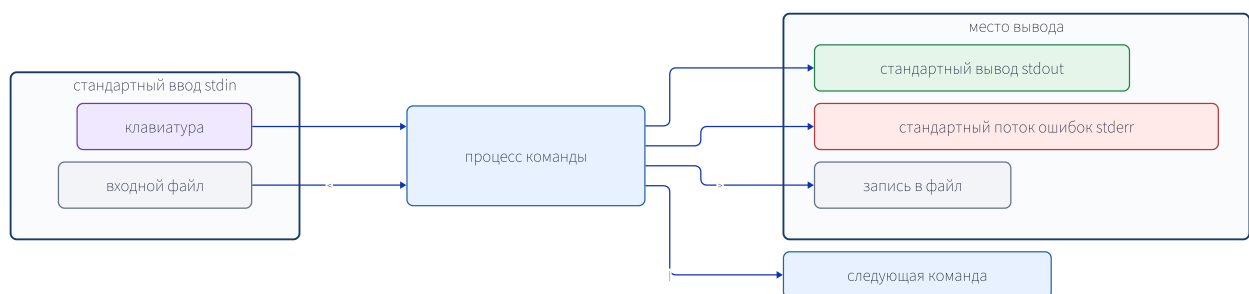
Рисунок 5-1. Три стандартных потока программы. > обычно направляет stdout в файл, а | соединяет stdout команды слева со stdin команды справа.
