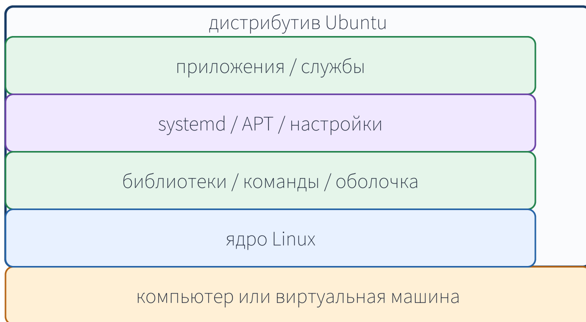
Рисунок 2-2. Дистрибутив объединяет ядро Linux, библиотеки, базовые команды, системное управление, пакеты и приложения. Ubuntu и Linux не следует считать полными синонимами.
