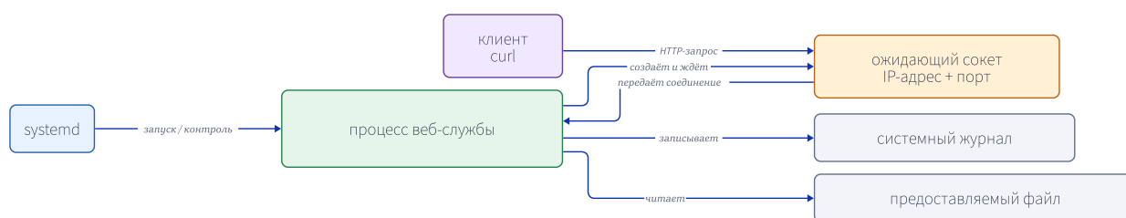
Рисунок 11-1. Управление ( systemd ), выполнение (процесс), сетевой механизм (ядро и сокет) и запрос клиента — разные этапы. У службы может быть несколько сокетов или вообще не быть сетевого обмена.
