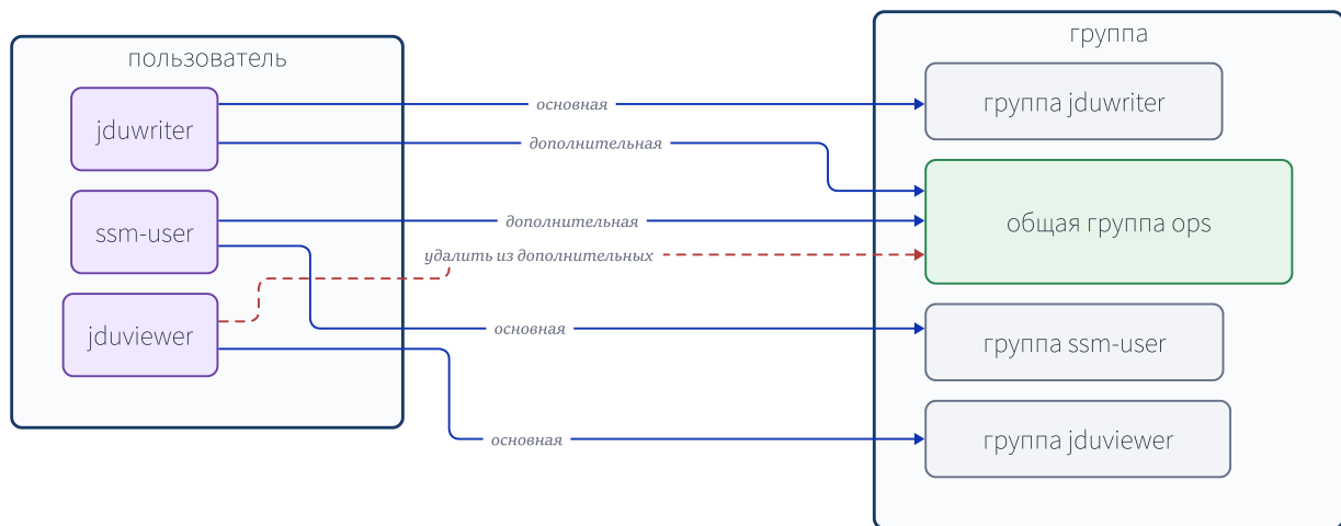
Рисунок 6-1. Связь основных групп пользователей с дополнительной группой для общих ресурсов.
