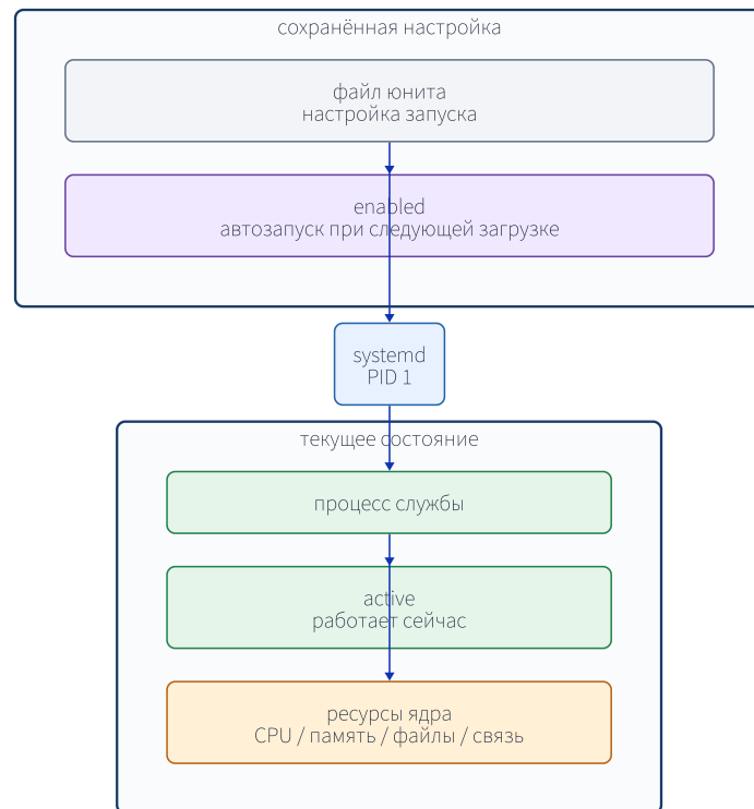
Рисунок 10-1. Юнит задаёт правила, systemd управляет, а процесс службы выполняет реальную работу.
