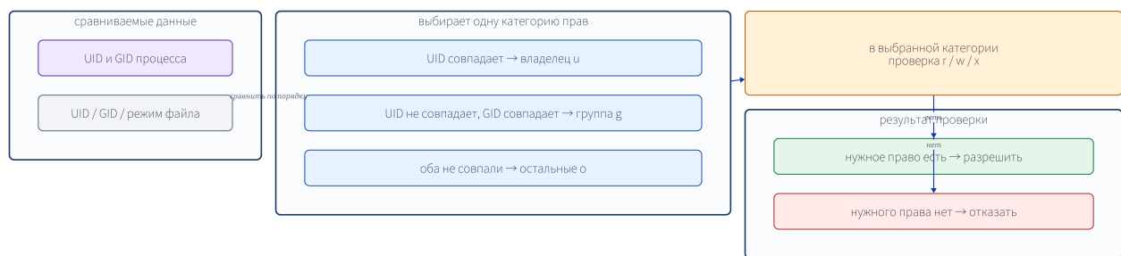
Рисунок 7-1. По учётным данным процесса выбирается категория u/g/o, затем её биты rwx определяют возможность действия.
