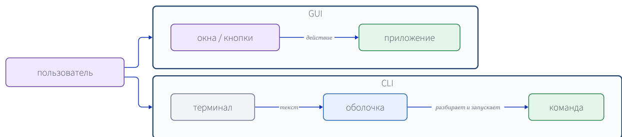
Рисунок 3-1. GUI и CLI — два способа взаимодействия; при использовании CLI важно различать терминал и оболочку.
