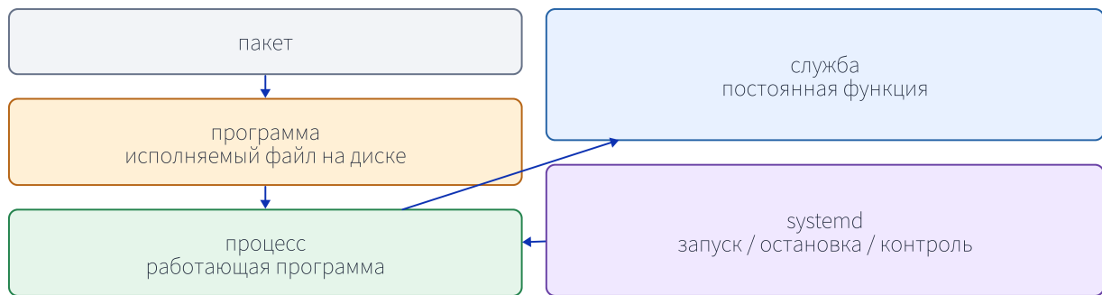
Рисунок 8-1. Различаем хранимую программу, работающий процесс, управляемую службу и распространяемый пакет.
