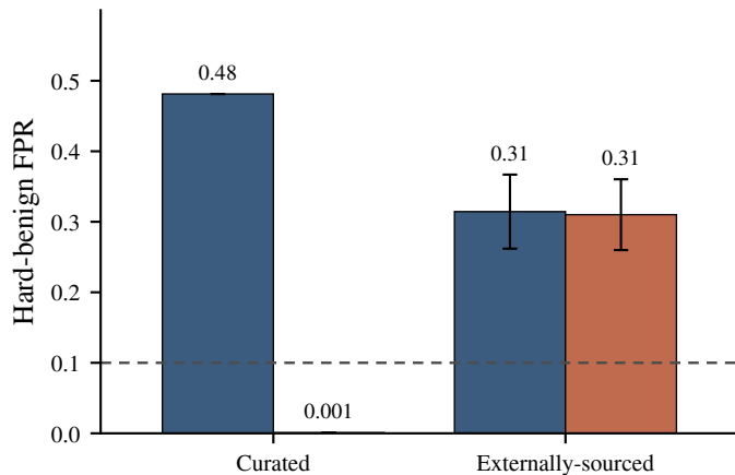
DeBERTa-v3-FT
