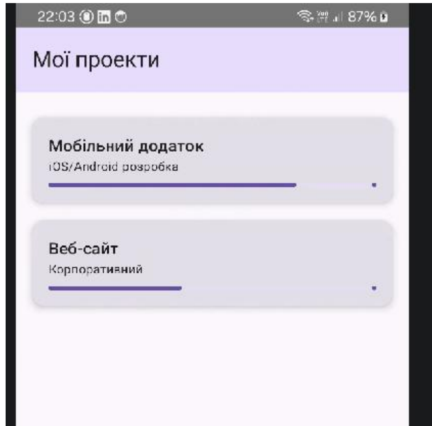
Рисунок 6 – Видалення проекту
