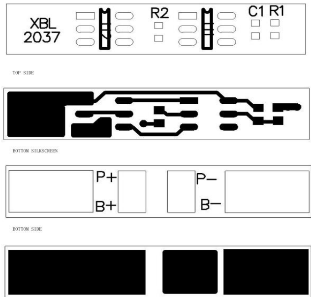
PCB 焊盘线路图及零部件名称规格表
