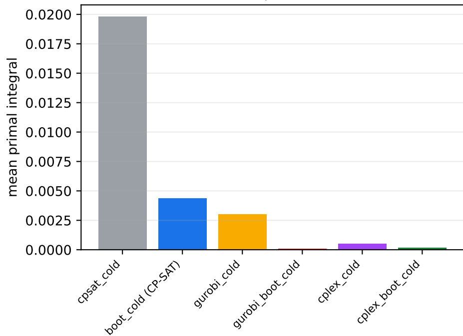
knapsack
