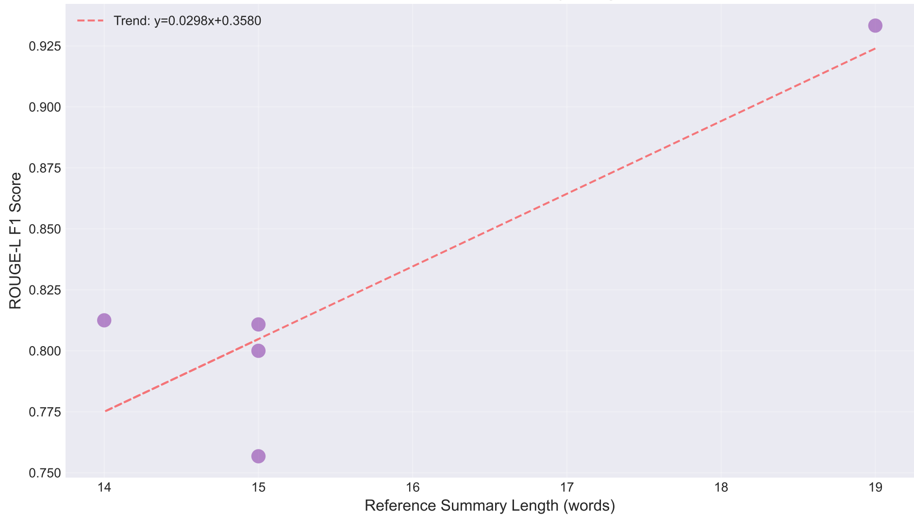
ROUGE-L F1 vs Summary Length
