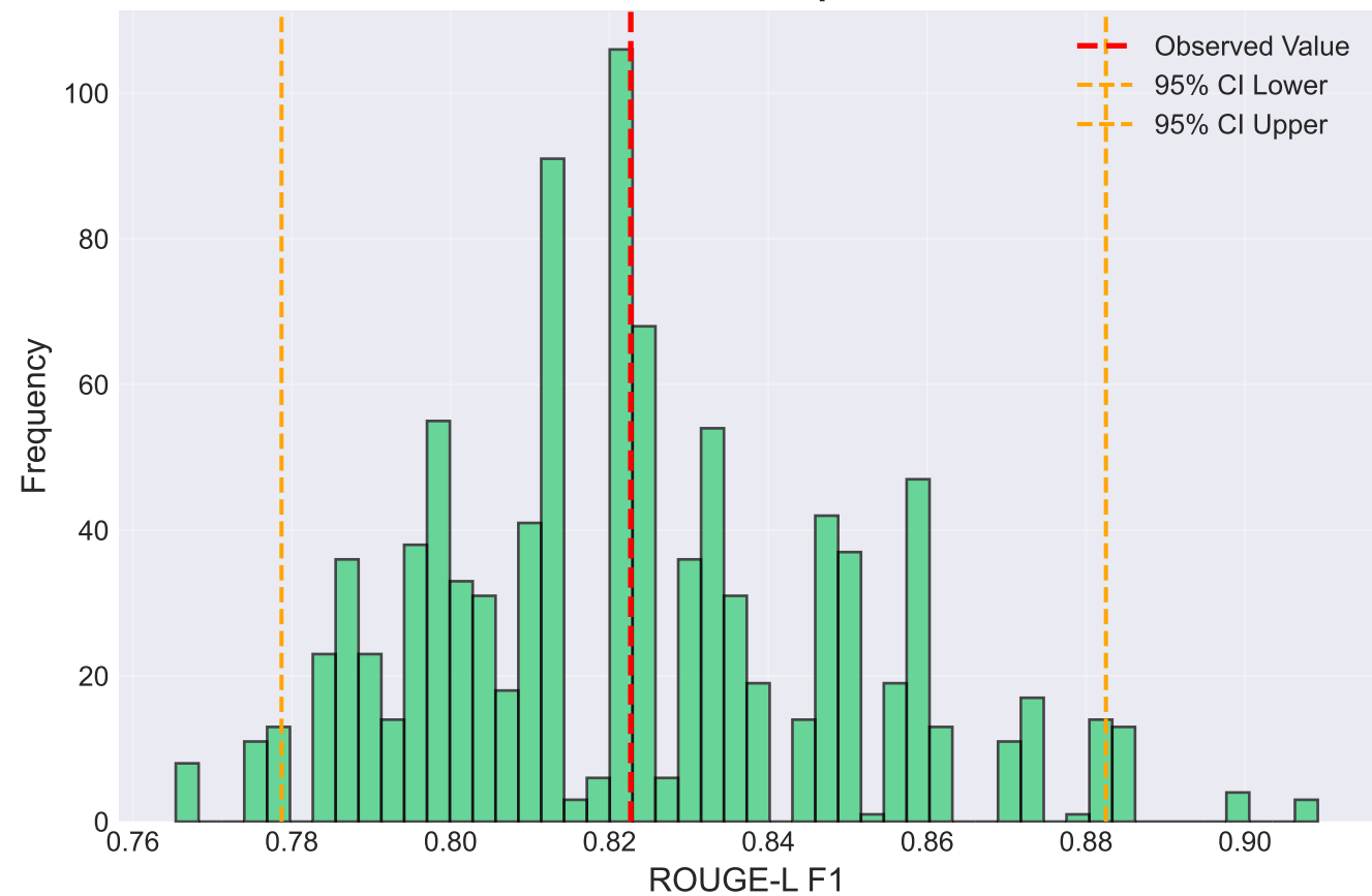
ROUGE-L F1 Bootstrap Distribution
