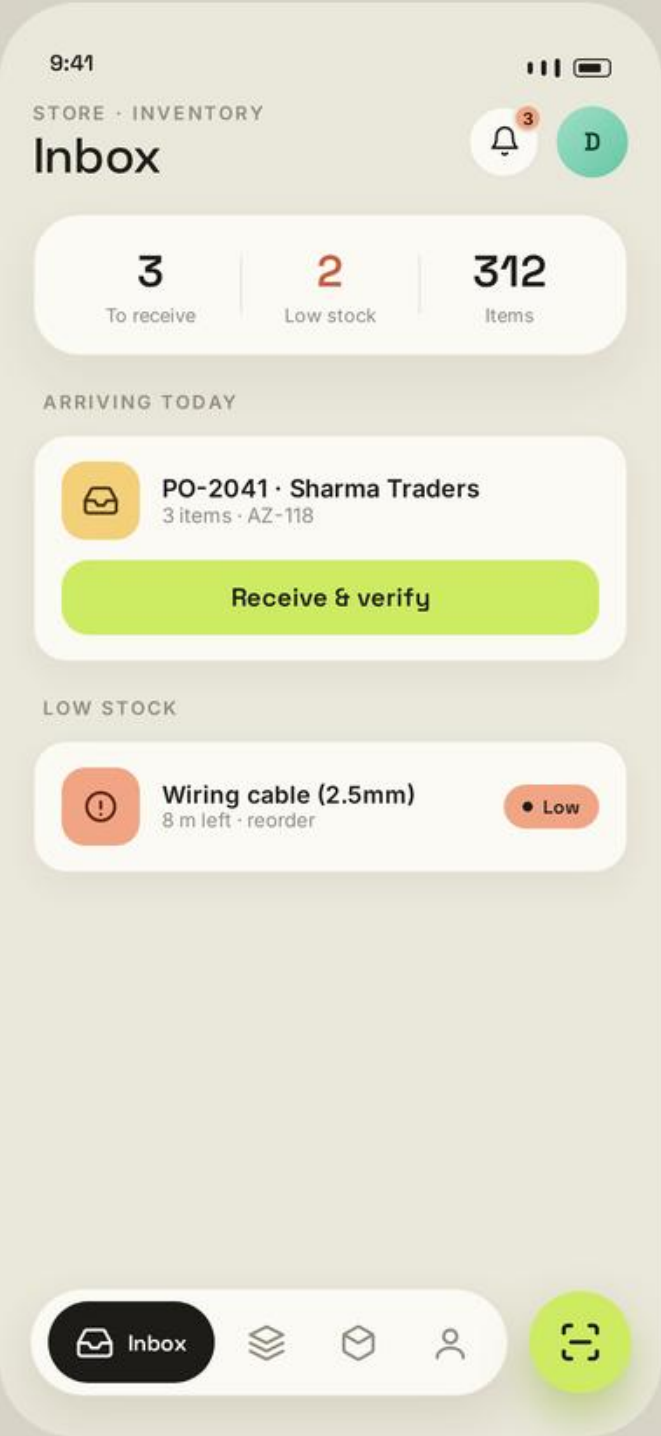
1. Inbox
