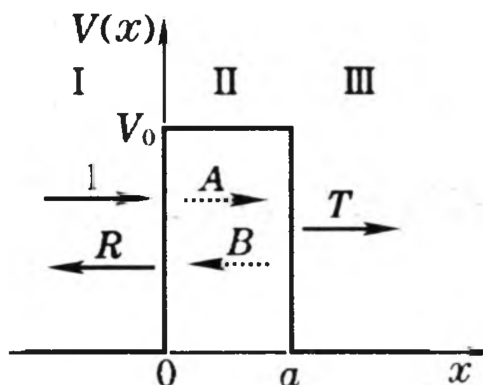
图 3.1: 一维方势垒
