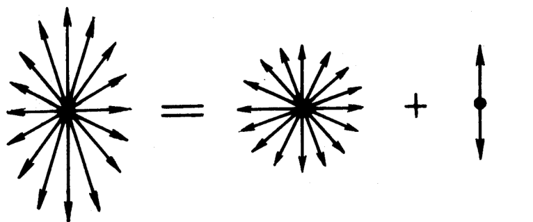
图 4.4: 部分偏振光透过检偏器
