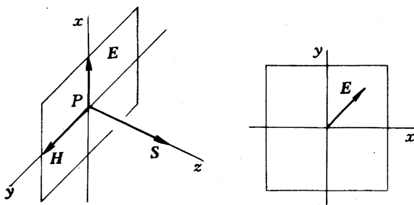
图 4.1: 光的偏振示意图
