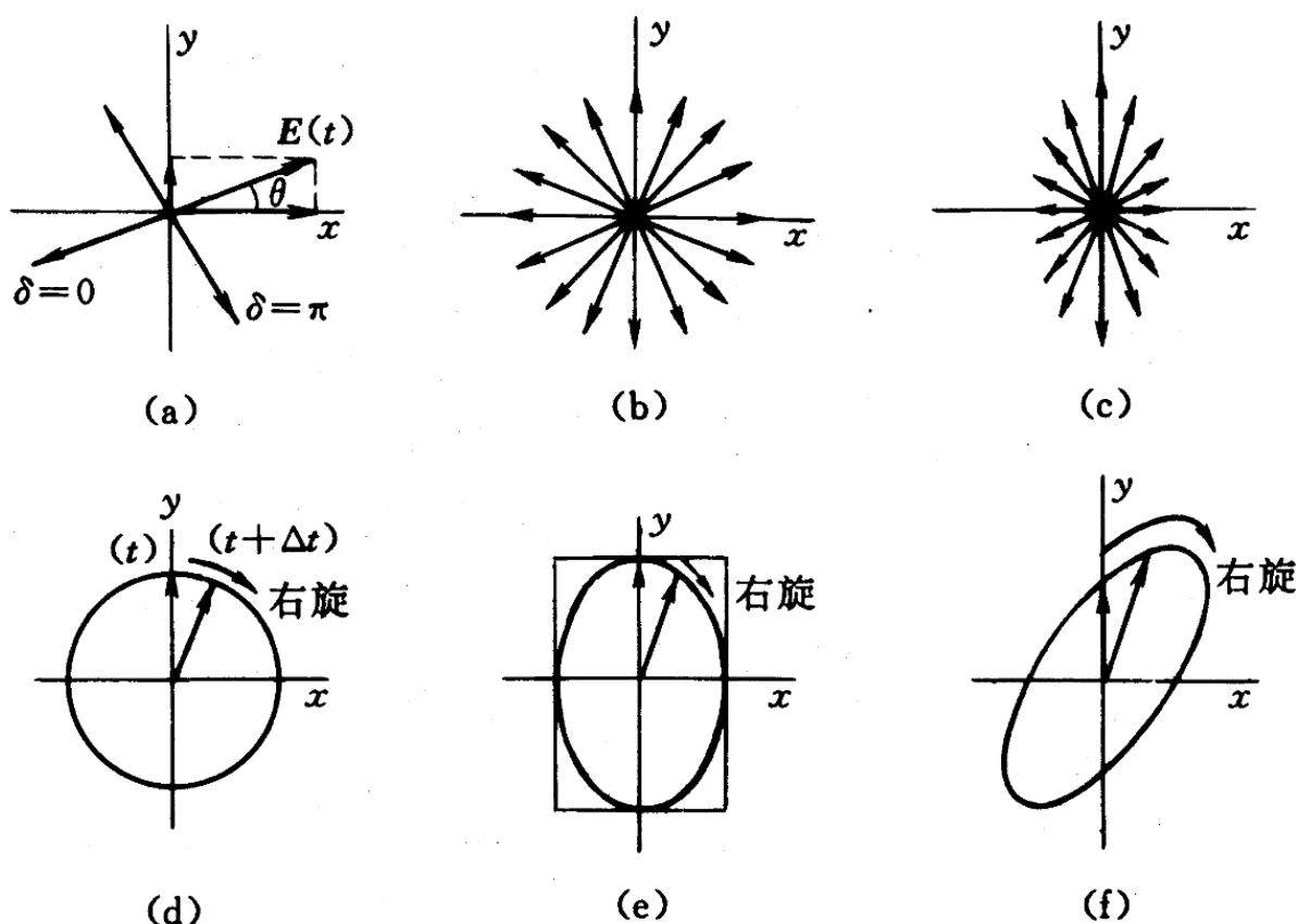
图 4.2: 光的五种宏观偏振态
