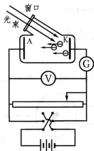
图 1.1: 光电效应实验装置
