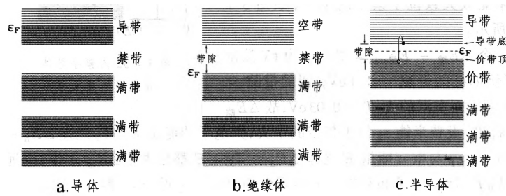
图 3.9: 三种导电材料的区别
