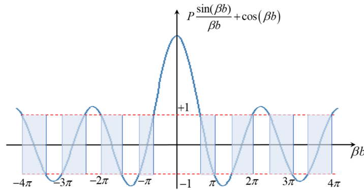
图 3.8: 允带与禁带
