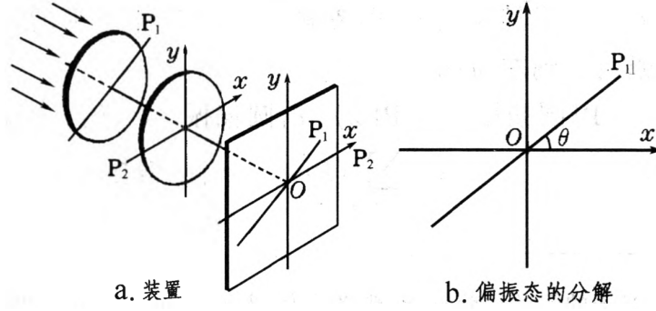
图 2.2: 线偏振态的分解
