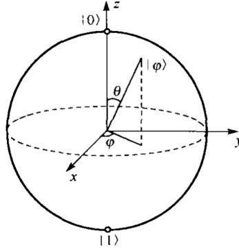
图 3.10: 布洛赫球
