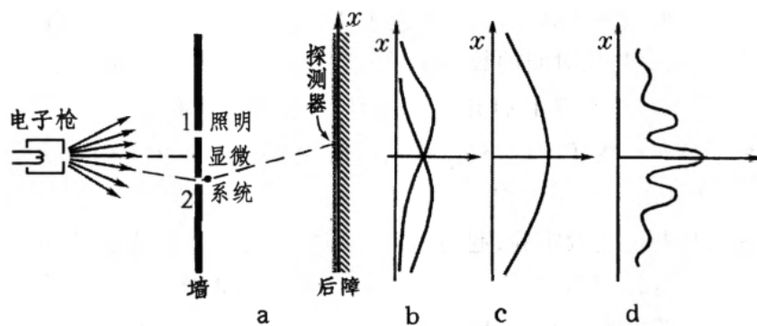
图 1.7: 追踪电子
