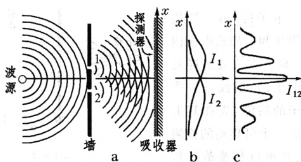
图 1.5: 经典波干涉
