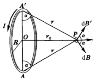
图 2.3: 圆线圈轴线上的磁场
