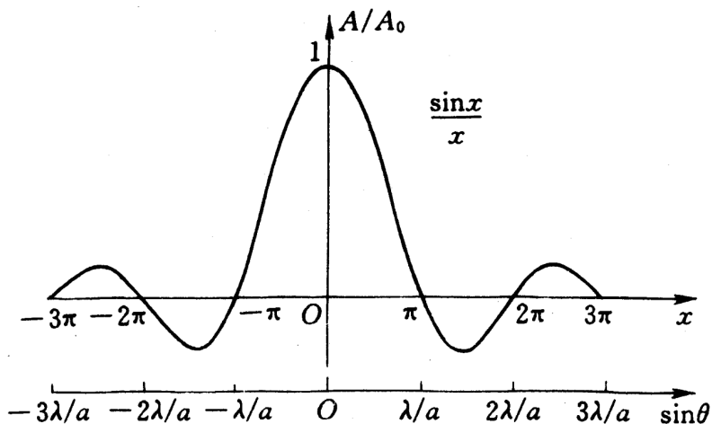
图 3.8: \text{sinc}(x) 图象
