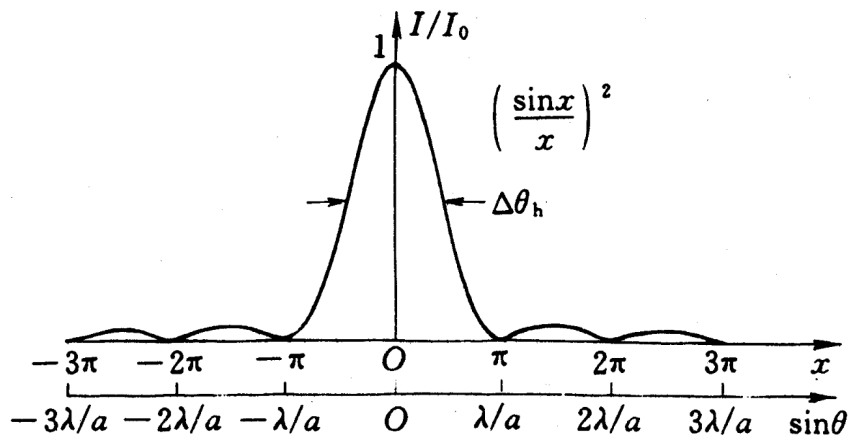
图 3.9: \text{sinc}^2(x) 图象
